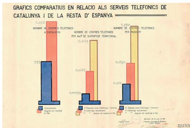
Gràfic sobre els centres telefònics a Catalunya i a Espanya, signat per l’enginyer Victorià Muñoz i Oms el 30 de juny de 1936. Fons Generalitat de Catalunya (Segona República). CAT/ANC 1-001 doc05-09 (imatge 148723).
