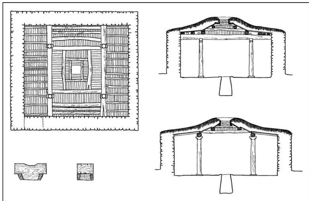
План перекрытый глхатуна , село Мартирос (Вайоц-дзор). Начало XX в. Архив ИАЭ. Папка 7. Чертежи Н. Папухяна
