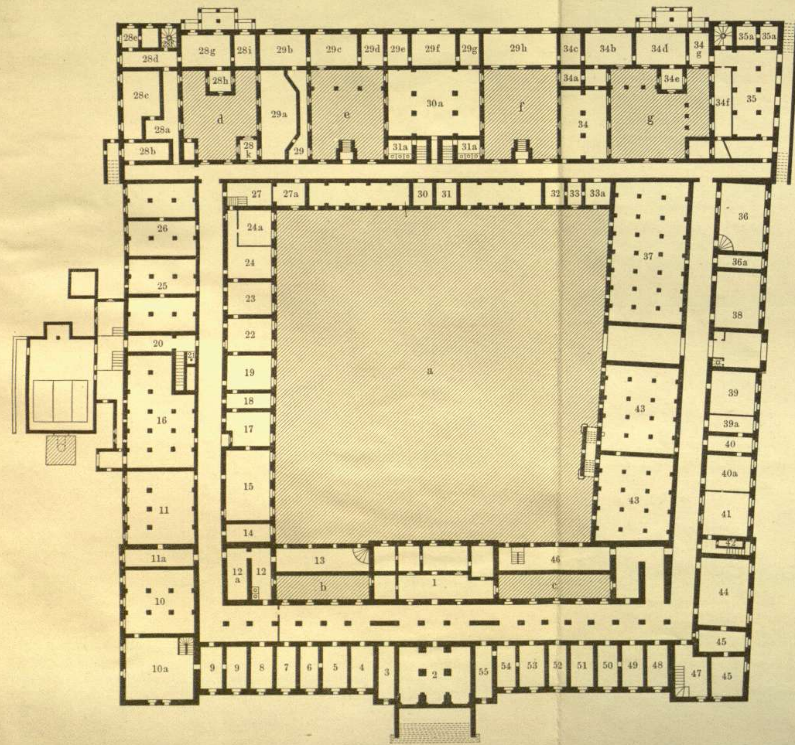
Kellergeschoß.
