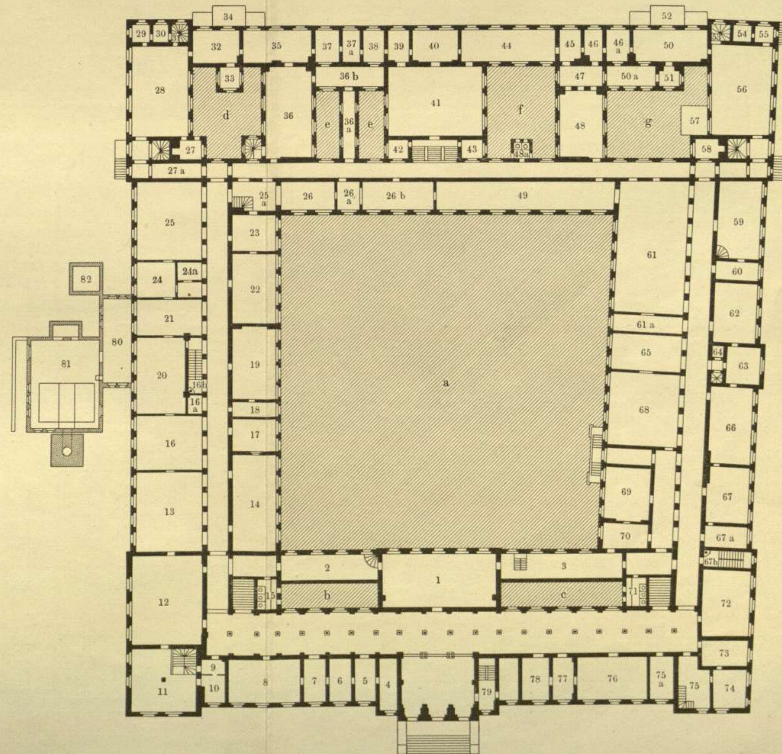
Erstes Geschoß.
