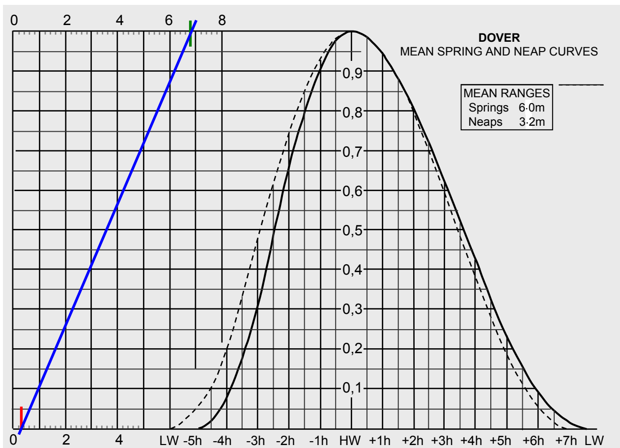
Abb. Tidenkurve von Dover mit (hier blau) eingezeichnetem Tidenstieg
