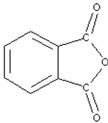
Anhidrido Ortoftálico
