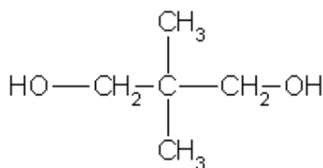
Neopentilglicol
