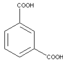
Acido Isoftálico
