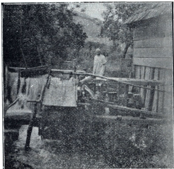
Piuă din Valea Zăgrii (Foto I. Morariu)
