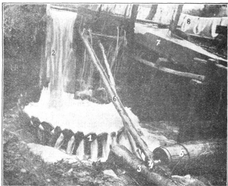
O »vâltoare« în asamblul ei. 1. Vâltoarea; 2. Șghiabul vâltorii (cu apă); 3. căpătai; 4. Cepul pe perinuță; 5. Grindeiul; 6. Cioroiu; 7. Șghiabul piuălor; 8. pânuri întinse pentru uscat.
