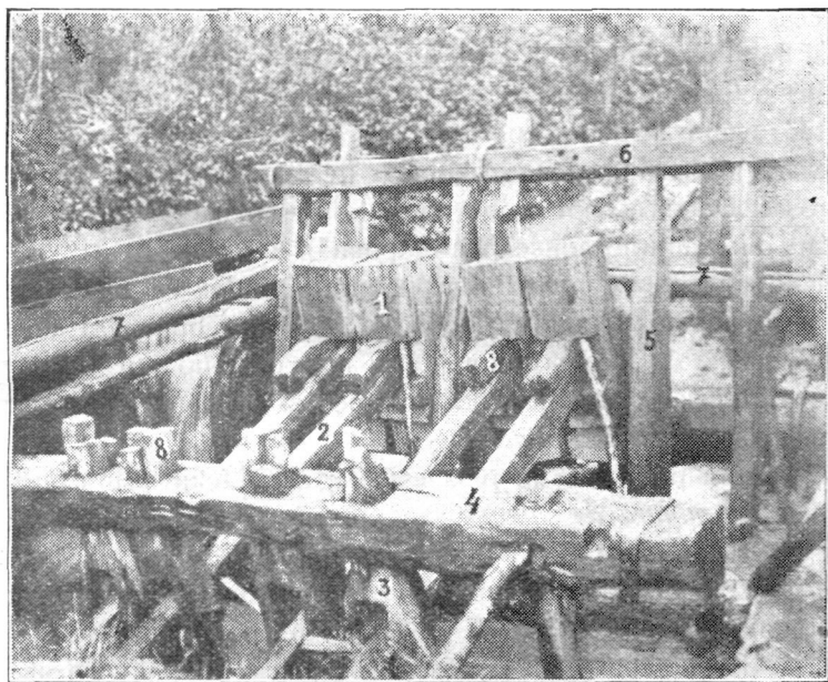
Vederea piuălor. 1. Pilug; 2. Tânel; 3. Urs; 4. Grinda dinapoi (a urșilor); 5. Spătare; 6. Grinda piuălor; 7. Cioroiu; 8. Icuri (găvoazde). (Foto I. Morariu)
