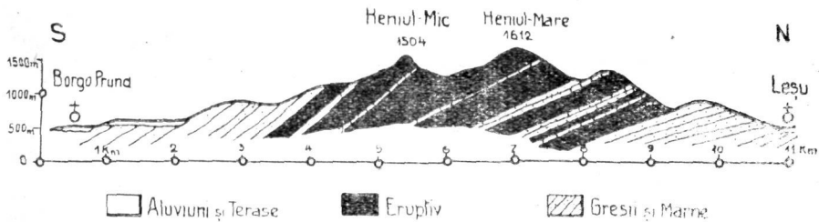
Profilul geologic al Muntelui Heniu.
