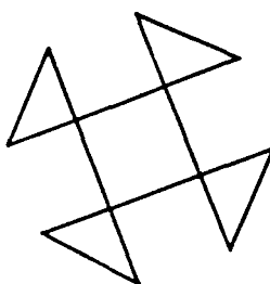
График последовательности 6), считанной по НКРТМВД
