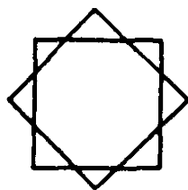
График ДЛПТВВ, считанной по НКРТМВД
