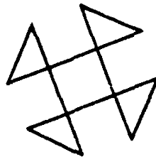
Алгоритм взаимопреобразования КРТФС в ВКРТМВД
