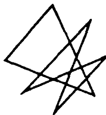
Алгоритм взаимопреобразования ВКРТМВД в КРТВВ
