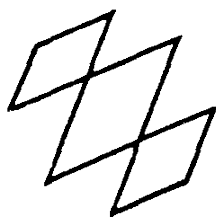
График ДЛПТВВ, считанной по КРТФС
