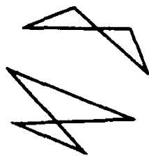
График ДЛПТВВ, считанной по КРТВВ
