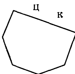
График последовательности 5), считанной по НКРТМВД
