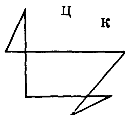
График последовательности 4), считанной по НКРТМВД
