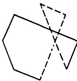
График реконструктивно дополненной последовательности 5), считанной по НКРТМВД
