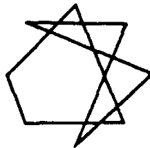
Алгоритм взаимопреобразования КРТФС в КРТВВ
