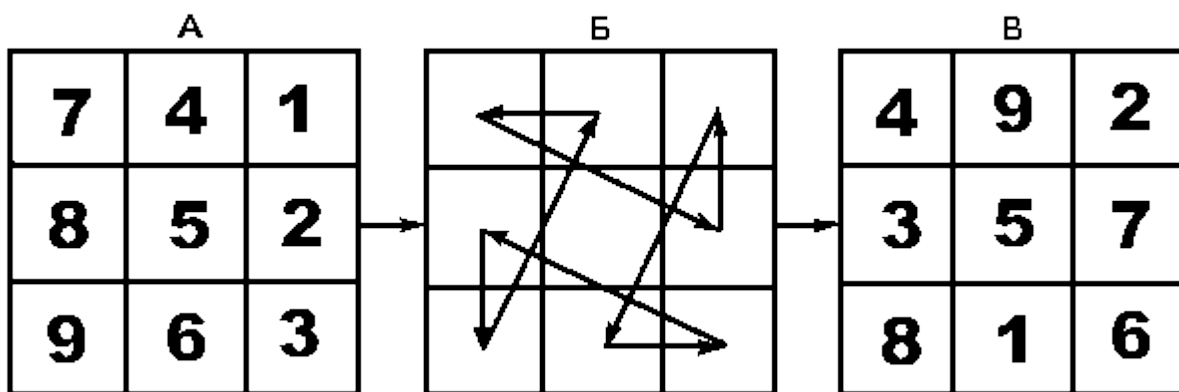
Алгоритм построения Ло шу
