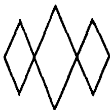
График ДЛПТВВ, считанной по ВКРТМВД
