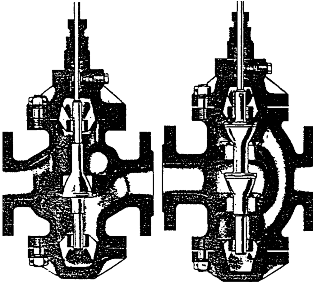
A seggio singolo
