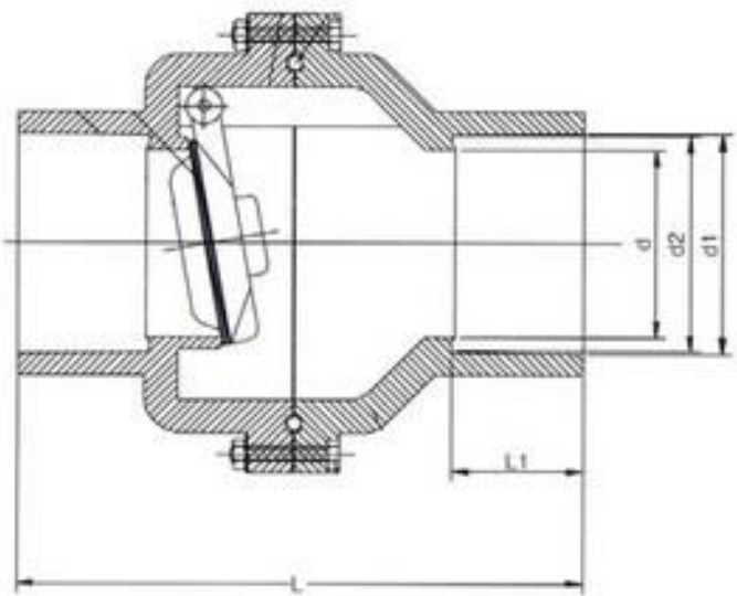
Valvola non ritorno
