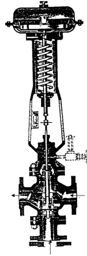
Testata inversa (Se manca l'aria chiudo la via diretta e apro la via squadra) 28
