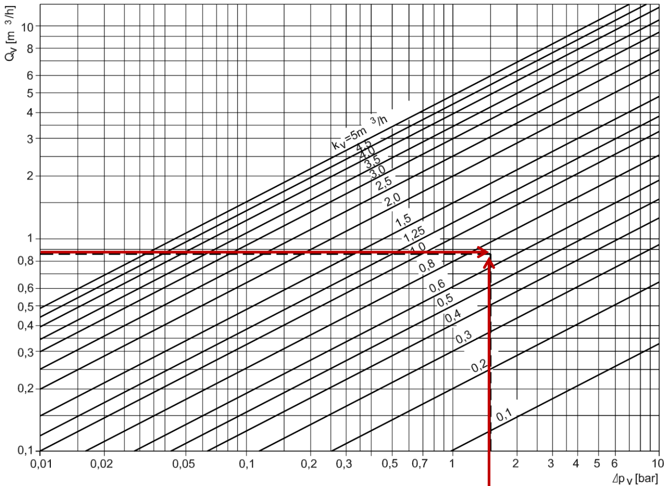
Fig. 2 Relazione tra quantità d'acqua e caduta di pressione nella valvola
