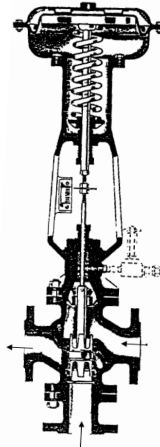
Testata diretta (Se manca l'aria apro la via diretta e chiudo la via squadra)
