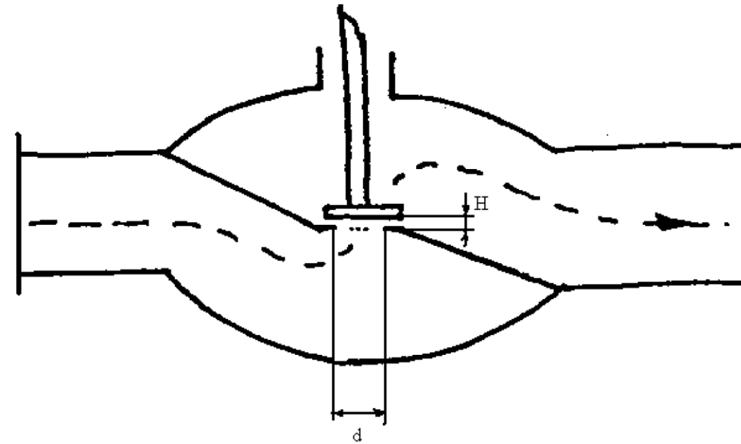
Valvola a flusso avviato
