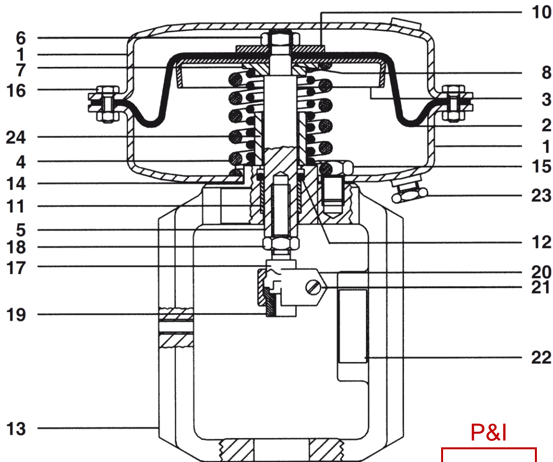
Servomotore PN4000
