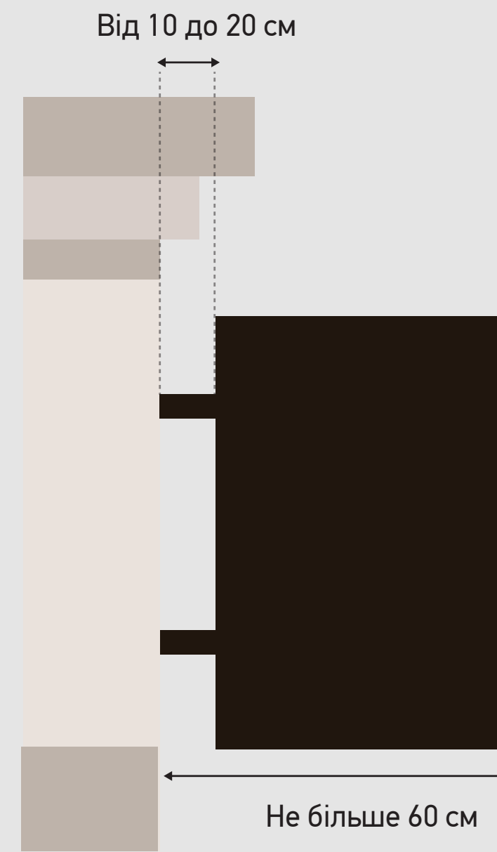
Вертикальна вивіска з подвійним кріпленням
