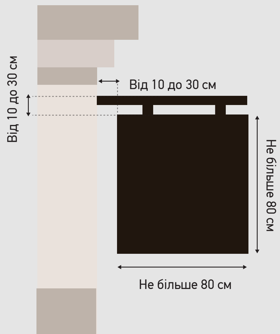
Підвісна вивіска з одним кріпленням
