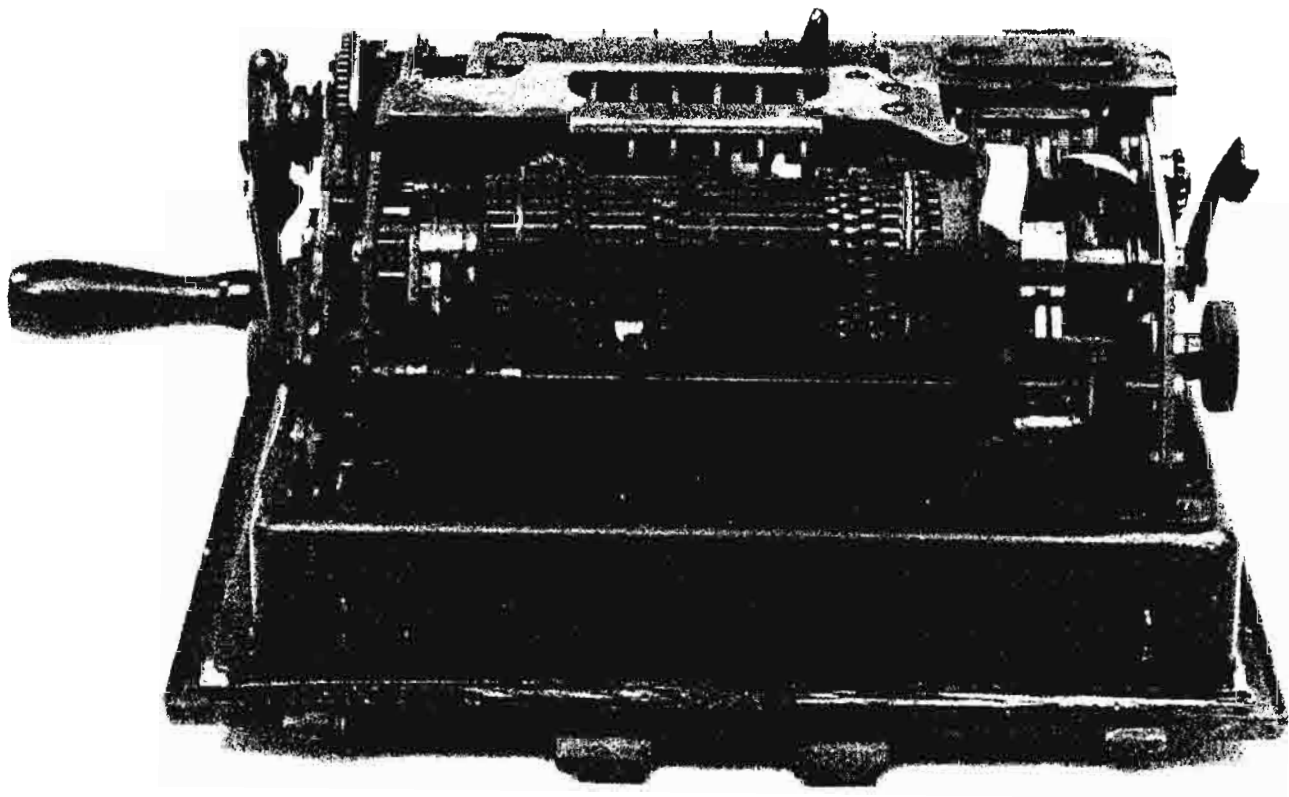
Fig. 3. Schlüsselerät 41. Rear view.
