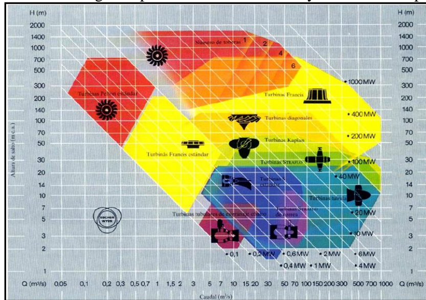
Gráfico No 1 Nomograma para selección de turbina y estimación de potencia
