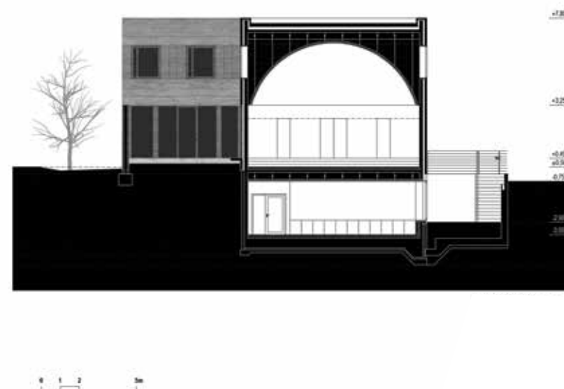
PRIKAZ 25 POPREČNI PRESJEK / ПРИКАЗ 25 ПОПРЕЧЕН ПРЕСЕК
