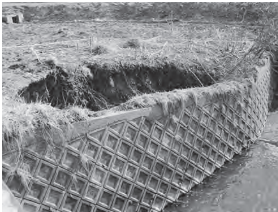
小徳明川護岸崩落状況 (9m)
