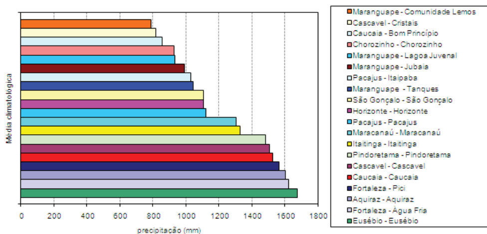
Figura 1 – Gráfico da Média Climatológica dos Postos Pluviométricos da RMF
