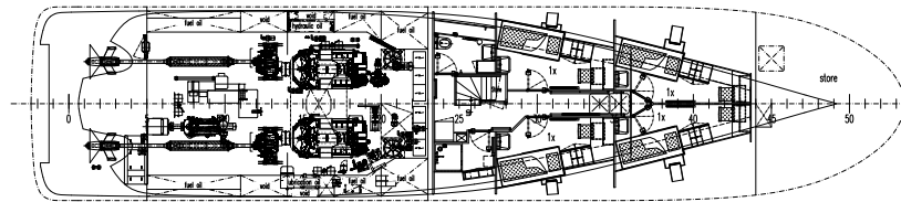
MAINDECK / TWEENDECK
