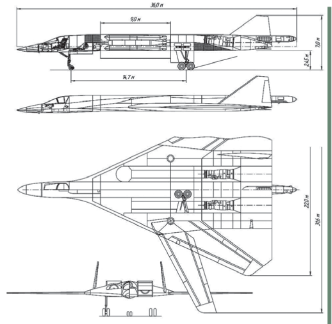
3. KÉP A PAK DA HÁROMNÉZETI RAJZA
