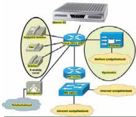
12. ÁBRA NEMZETI VSAT-RENDSZER VÉGPONTI ARCHITEKTÚRÁJA (FORRÁS: A SZERZŐK ARCHÍVUMA, EGYÜTTMŰKÖDÉSBEŒN A HUNGARO DIGITEL KFT.-VEL)
