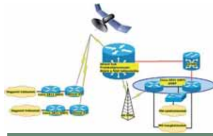
11. ÁBRA NEMZETI VSAT-RENDSZERVÁZLAT (FORRÁS: A SZERZŐK ARCHÍVUMA, EGYÜTTMŰKÖDÉSBEŒN A HUNGARO DIGITEL KFT.-VEL)
