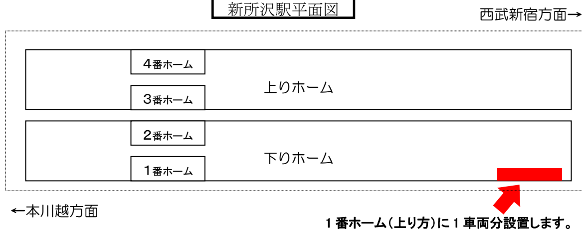
新所沢駅平面図
