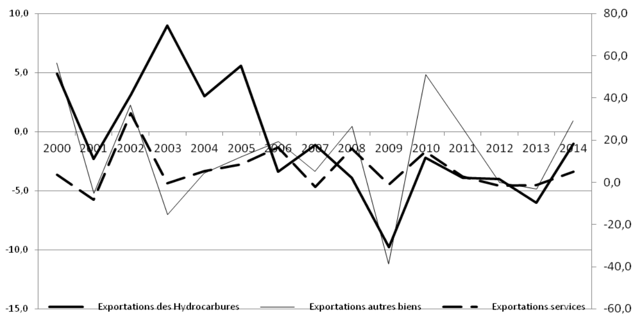
Evolution en volume des exportations de biens et services (en %) Echelle de droite : Autres biens et services. Echelle de gauche : Hydrocarbures
