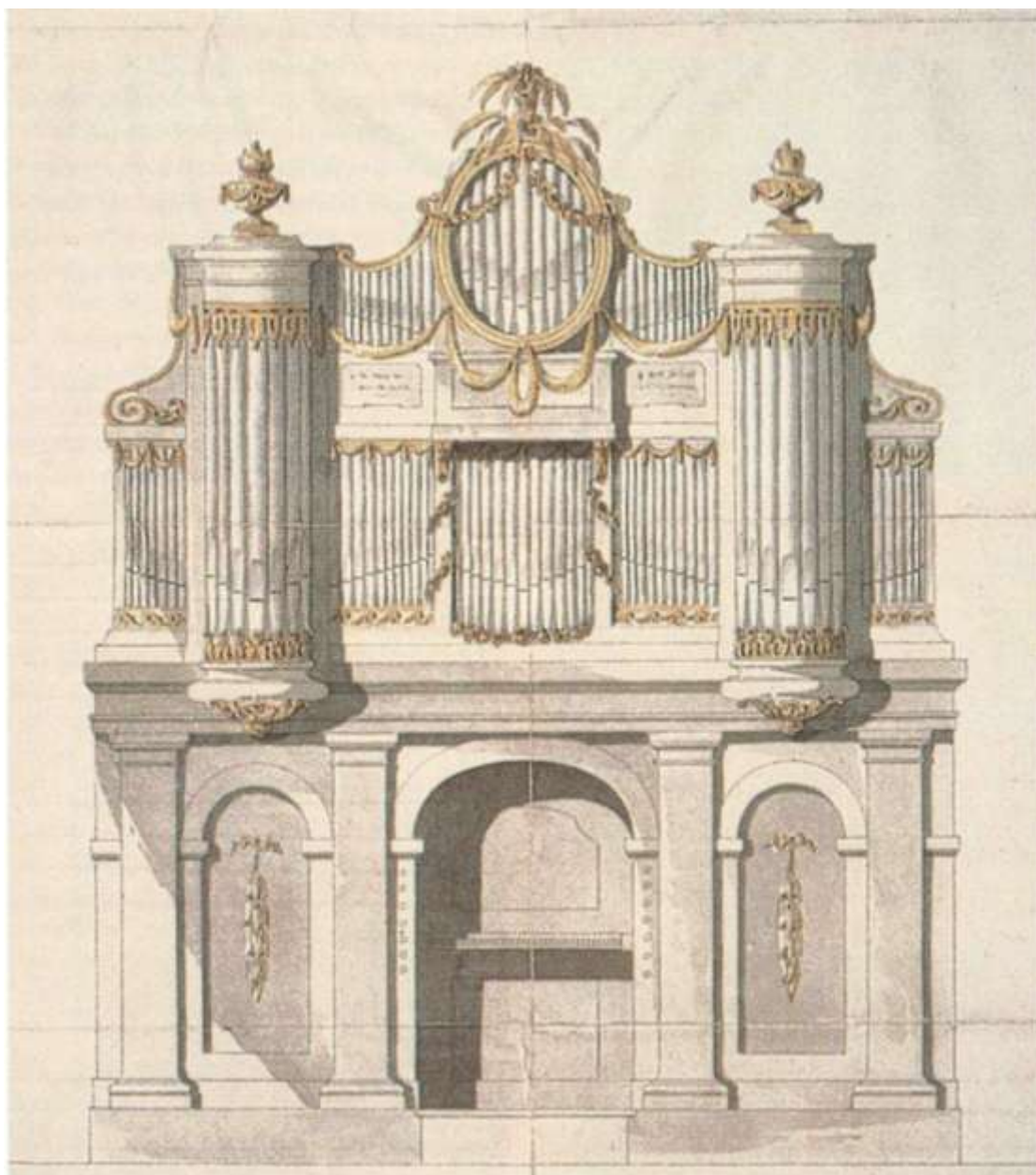
Ritning till orgelfasad av Olof Tempelman för orgel av Lars Strömblad till Kärna kyrka. Efter Tempelman – Arkitekten Olof Tempelman 1745–1816 av Lena Berg Villner (Västervik 1997 s. 196). Jämför den bevarade fasaden från 1784 års orgel av Strömblad i Rogslösa kyrka, se foto ovan.
