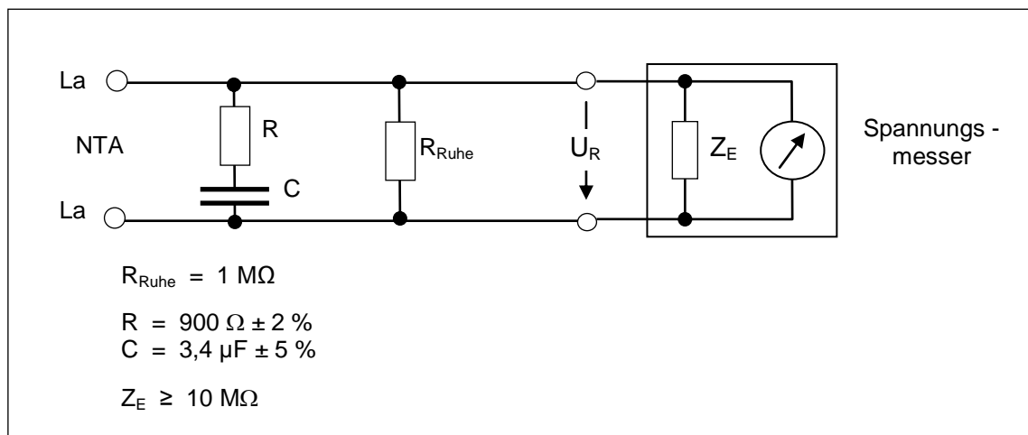
Abbildung Anhang D- 4 : Messung der Anruf-Gleichspannung
