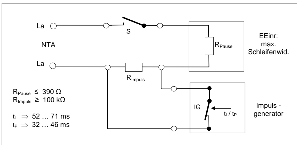
Abbildung Anhang D- 5 : Auswertung der IWV- Wählzeichen
