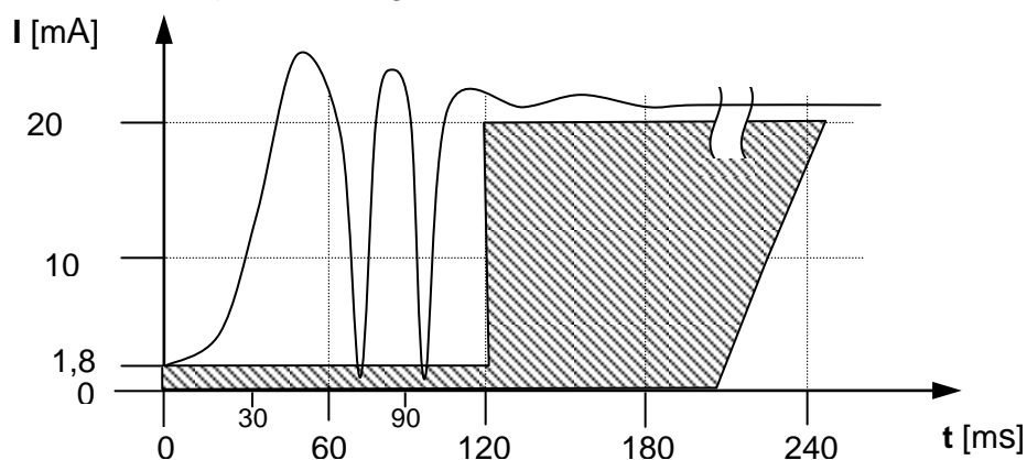
Abbildung 6-1 : Belegungs-Einschwingdauer
