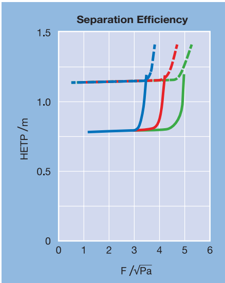
Mellapak 125.Y Mellapak 125.X 960 ——— 960 - - - - 100 ——— 100 - - - - 50 ——— 50 - - - - parameter = head pressure p / mbar
