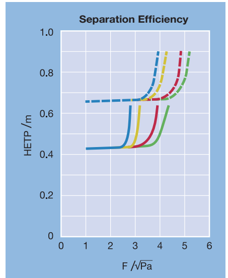
Mellapak 2Y Mellapak 2X 960 ——— 960 - - - - 400 ——— 400 - - - - 100 ——— 100 - - - - 50 ——— 50 - - - - parameter = head pressure p / mbar
