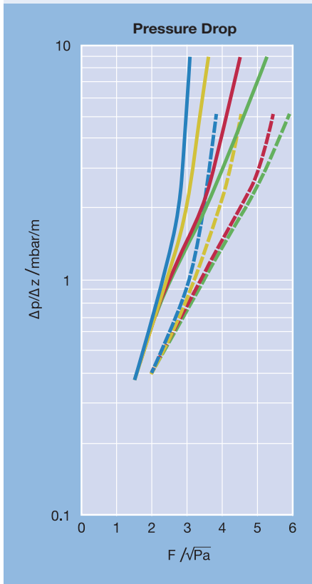
Mellapak 170.Y Mellapak 170.X
