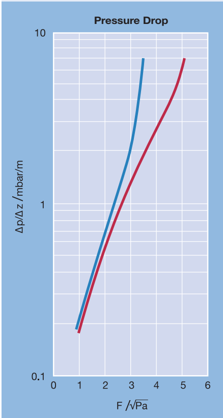
MellapakPlus 202.Y
