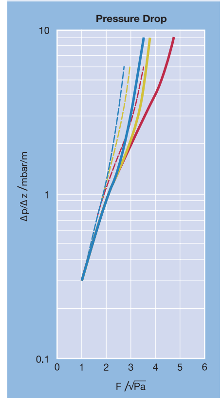
MellapakPlus 252.Y vs. Mellapak 250.Y
