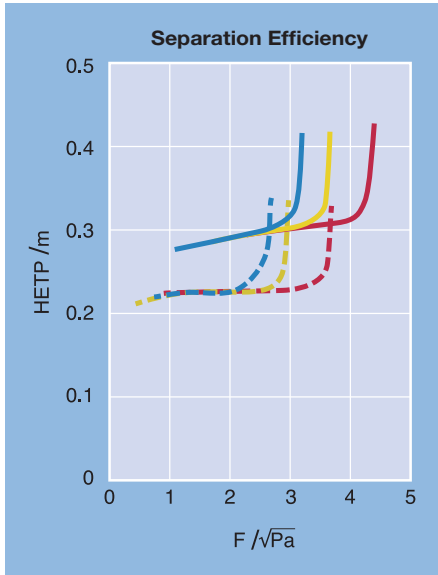
MellapakPlus 352.Y MellapakPlus 602.Y 960 ——— 960 - - - 400 ——— 400 - - - 100 ——— 100 - - - parameter = head pressure p /mbar
