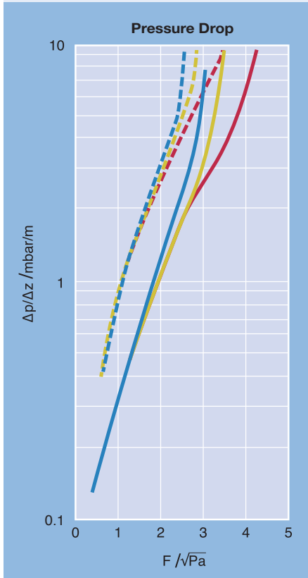
MellapakPlus 352.Y MellapakPlus 602.Y
