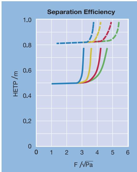
Mellapak 170.Y Mellapak 170.X 960 ——— 960 - - - - 400 ——— 400 - - - - 100 ——— 100 - - - - 50 ——— 50 - - - - parameter = head pressure p / mbar
