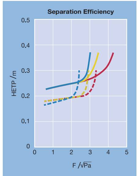
MellapakPlus 452.Y MellapakPlus 752.Y 960 ——— 960 - - - 400 ——— 400 - - - 100 ——— 100 - - - parameter = head pressure p /mbar
