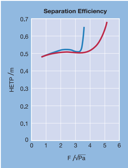
MellapakPlus 202.Y 960 ——— 100 ——— parameter = head pressure p /mbar
