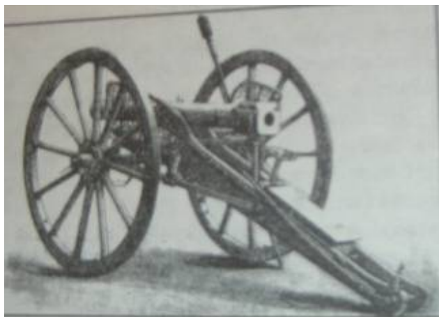
Tun „Krupp” calibru 78,5 mm, model 1868 1
