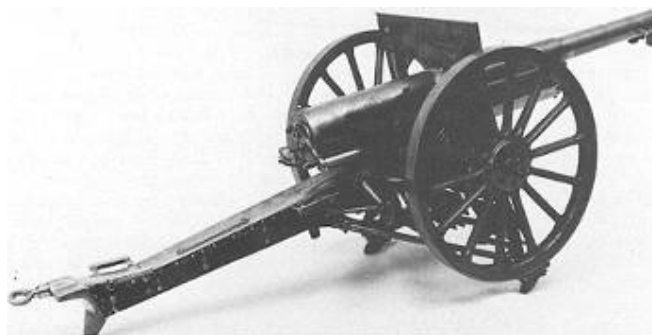
Tunul divizionar de câmp „Schneider” cal. 75 mm md.1897 Sursa: Richard A. Gabriel, Karen S. Metz, A SHORT HISTORY OF WAR The Evolution of Warfare and Weapons.
