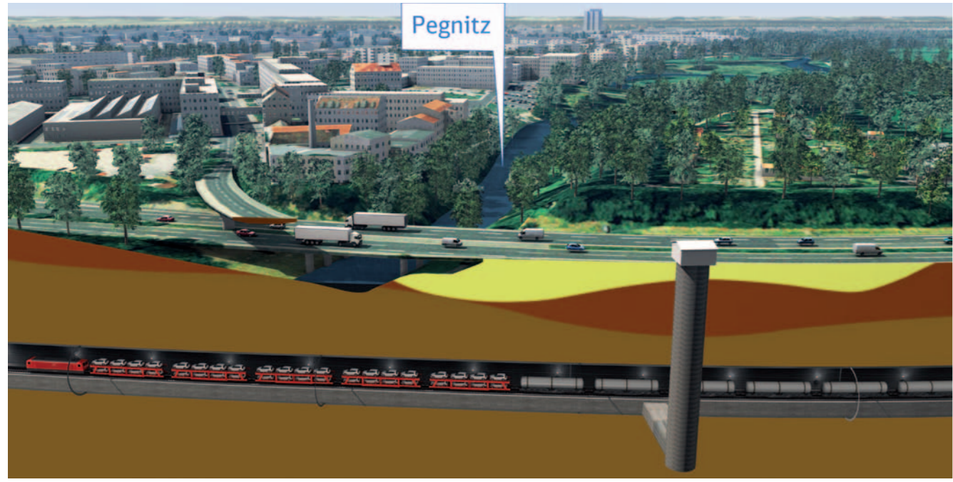
Güterzugtunnel (Visualisierung)
