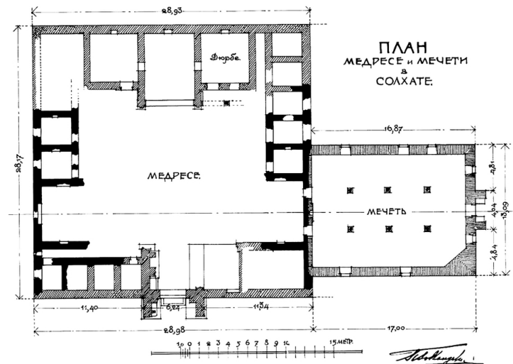
План медресе и мечети в Солхате. Чертеж П.И. Голландского. 1926.
