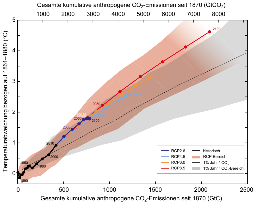
Abbildung SPM.10 | Anstieg der mittleren globalen Erdoberflächentemperatur als Funktion der kumulativen totalen globalen CO 2 -Emissionen aus verschiedenen Anhaltspunkten. Multimodell-Resultate von einer Hierarchie von Klima-Kohlenstoffkreislauf-Modellen für jeden RCP bis 2100 sind mit farbigen Linien und Jahrzehnt-Mitteln (Punkte) dargestellt. Einige Jahrzehnt-Mittel sind zur besseren Übersichtlichkeit angegeben (z.B. 2050 für das Jahrzehnt 2040–2049). Die Modellresultate für den historischen Zeitraum (1860 bis 2010) werden in Schwarz angezeigt. Die farbige Fahne illustriert den Multimodell-Streubereich über die vier RCP-Szenarien und verblasst mit der abnehmenden Zahl der für RCP8.5 verfügbaren Modelle. Das von CMIP5-Modellen simulierte Multimodell-Mittel und die entsprechende Bandbreite, angetrieben durch einen CO 2 -Anstieg von 1% pro Jahr (1%-pro-Jahr-CO 2 -Simulationen), werden durch eine dünne schwarze Linie und eine graue Fläche wiedergegeben. Für eine spezifische Menge von kumulativen CO 2 -Emissionen ergeben die 1%-pro-Jahr-CO 2 -Simulationen eine geringere Erwärmung als die, die durch RCPs getrieben werden, welche zusätzliche Nicht-CO 2 -Antriebe einbeziehen. Die Temperaturwerte beziehen sich auf den Basiszeitraum von 1861–1880, die Emissionen beziehen sich auf 1870. Jahrzehnt-Mittel sind durch gerade Linien verbunden. Für weitere technische Details siehe Zusatzmaterial der Technischen Zusammenfassung. {Abbildung 12.45; TS TFE.8, Abbildung 1}
