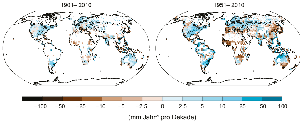
Abbildung SPM.2 | Karten der beobachteten Niederschlagsänderungen von 1901 bis 2010 und von 1951 bis 2010 (die Trends der jährlichen Akkumulation wurden unter Verwendung der gleichen Kriterien wie in Abbildung SPM.1 berechnet) von einem Datensatz. Für weitere technische Details siehe Zusatzmaterial zur Technischen Zusammenfassung. {TS.TFE.1 Abbildung 2; Abbildung 2.29}
