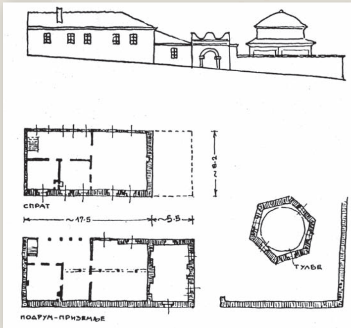
Турбе шеих мусџафе и Текија, црџеж Turbah of sheih Mustafa, drawing
