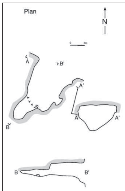
איור 15: מערה 348C, תוכנית וחתכים
