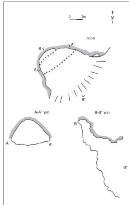
איור 5: תכנית וחתכים של מערת "לנחמ עבדי" (349)
