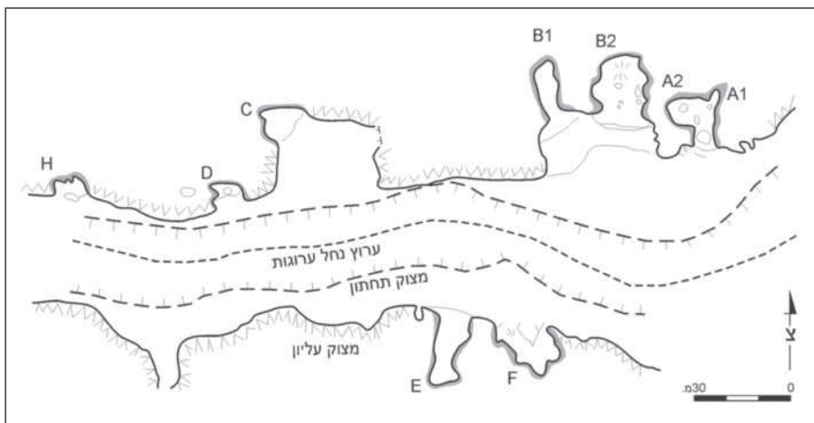
איור 17: תכנית מערות הנטיפים (304)
