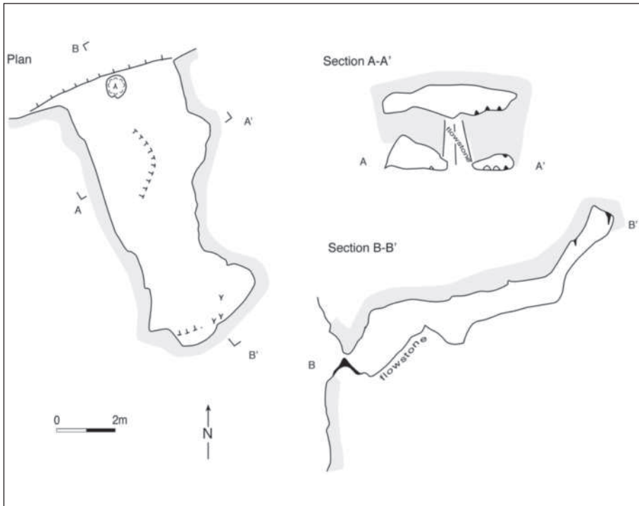
איור 20: מערה 304E, תוכנית וחתכים
