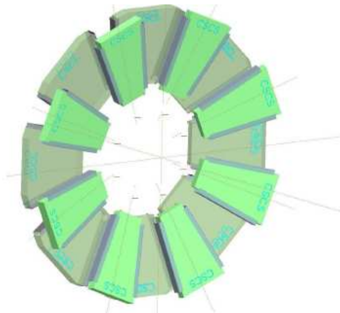
Рис.5.4. Размещение восьми больших и восьми малых камер CSC в торцевой части детектора ATLAS.
