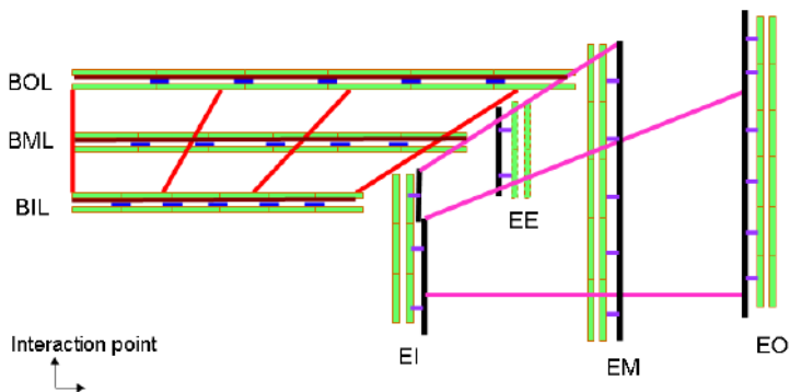
Рис.5.6. Общая схема позиционирования мюонного спектрометра ATLAS.
