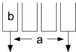
Рис.5.5 Схема считывания сигнала CSC камер. Ширина стрипа больших и малых камер составляет величину b = 1,519 и 1,602 мм, соответственно. Межстриповый промежуток 0,25 мм. Шаг электроники считывания a , соответственно, равен a = 5,308 и 5,567 мм. Наведенный сигнал считывается с катодных стрипов.
