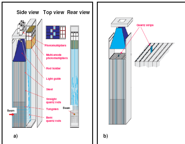
Рис.6.4. Схема модулей детектора ZDC.:a) электромагнитный модуль, в нижней части снаружи видны изогнутые координатные стержни, b) деталь, показывающая положение кварцевых стержней в бороздах (стрипах).
