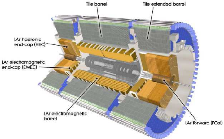
Рис.4.1. Система калориметров детектора ATLAS.
