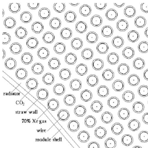
Рис.3.14. Схема расположения трубок в модуле центральной части Детектора переходного излучения. Между трубками расположено вещество радиатора. Трубки окружены оболочкой, заполненной газом \text{CO}_2 , предохраняющим объем внутри трубки от возможных загрязнений извне.
