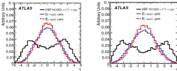
Рис.14.1.8а. Распределение по псевдобыстроте \eta струи с максимальным p_T (слева) и второй по величине p_T струи (справа) для сигнала (сплошная линия) и фоновых событий.
