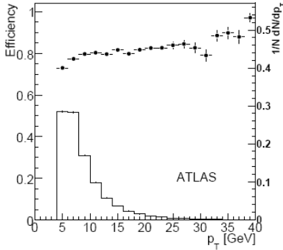
Рис.13.17. Эффективность реконструкции мюонов (левая шкала) и спектр поперечных импульсов мюонов (правая шкала) для распада B_s^0 \rightarrow \mu\mu . Триггер p_{T1(2)} \geq 6 (4) ГэВ/с.
