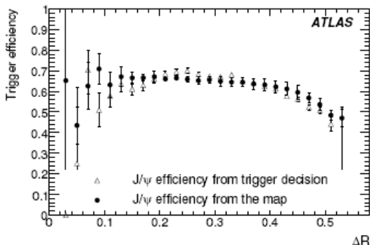
Рис.13.3. Полная эффективность триггера двух мюонов на J/\Psi в зависимости от \Delta R , радиуса RoI первого мюона L1.
