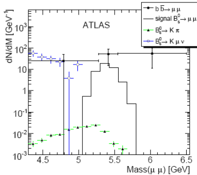
Рис.13.18. Распределения эффективных масс пар мюонов для сигнальных (гистограмма) и фоновых событий для распада B_s^0 \rightarrow \mu\mu . Количество событий соответствует интегральной светимости 10 \text{ фб}^{-1} .
