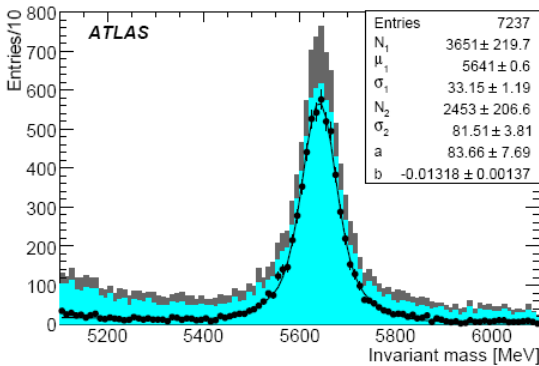
Рис.13.15. Распределения эффективных масс \mu\mu . Точками показано распределение после применения всех критериев отбора.
