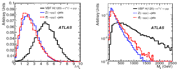
Рис.14.1.86. Распределение по величин интервала псевдобыстроты \Delta\eta (слева) между струями с максимальными p_T и по эффективной массе этих двух струй (справа) для тех же событий.
