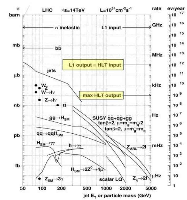
Рис.8.1. Сечения (левая шкала) и скорости потока соответствующих событий (шкала справа) различных физических процессов pp -взаимодействий при энергии и светимости LHC 14 ТэВ и 10^{34}\text{cm}^{-2}\text{s}^{-1} .
