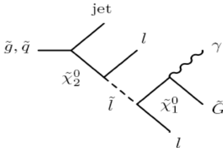
Рис.15.7. Диаграмма распада самого легкого нейтралино NLSP \tilde{\chi}_1^0 на гравитино \tilde{G} и фотон. Процесс возможен в модели GMSB с N=1 и малой величиной \tan\beta , когда нейтралино
