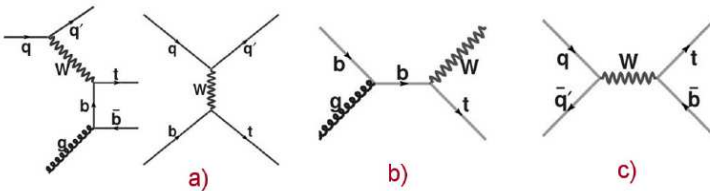
Рис.12.3. Диаграммы трех механизмов одиночного рождения t -кварка в лидирующем порядке теории возмущений КХД: t -канальный; W_t – ассоциированное рождение и s -канальный.
