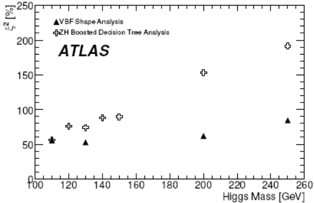
Рис.14.2.12. Чувствительность наблюдения невидимого распада бозона Хиггса для случаев VBF (темные символы) и ZH рождения (открытые символы) для 30 \text{ fb}^{-1} на уровне достоверности 95%. Учтен фон Стандартной модели и систематические погрешности. Величина чувствительности \xi^2 определена как число сигнальных событий, необходимых, чтобы увеличить полное количество событий (счет) на фактор, в 1,64 раза превышающий неопределенность в числе фоновых событий:
