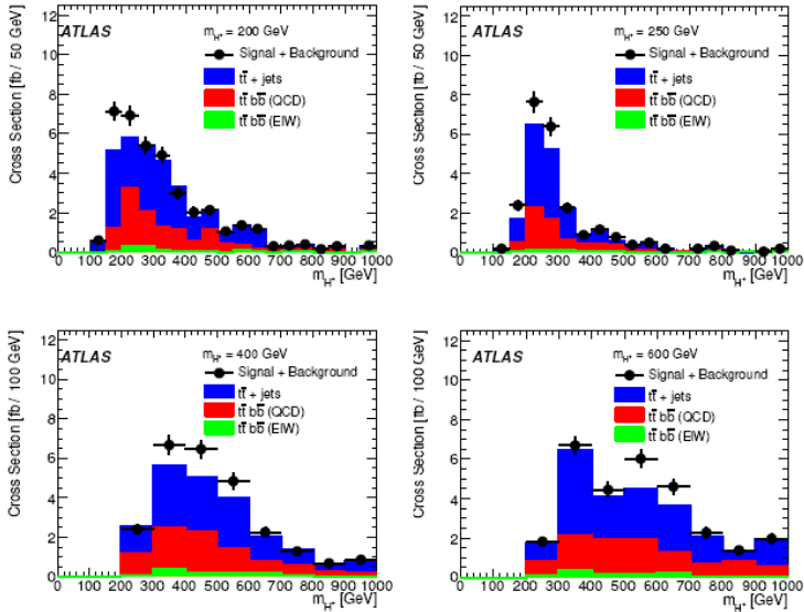
Рис.14.2.17. Реконструированные события сигнала и фона для масс H^+ 200, 250, 400 и 600 ГэВ в канале gg/gb \rightarrow t[b] H^+ \rightarrow t[b] tb \rightarrow bW[b]bWb \rightarrow b\ell\nu[b]bqqb . Пояснения см. текст.
