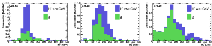
Рис.14.2.15. Распределения поперечных масс N_+ для канала gg/ gb \rightarrow t [b] H^+ \rightarrow bqq[b] \tau(\text{адр}) \nu для трех значений массы N_+ 170, 250 и 400 ГэВ. Фон соответствует значению \tan\beta = 35 .
