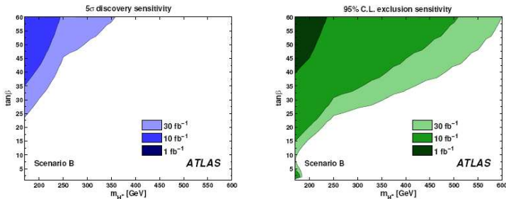
Рис.14.2.16. Ожидаемые результаты для открытия (слева) и контуры исключения для канала gg/ gb \rightarrow t [b] H^+ \rightarrow bqq[b] \tau(adp) \nu .
