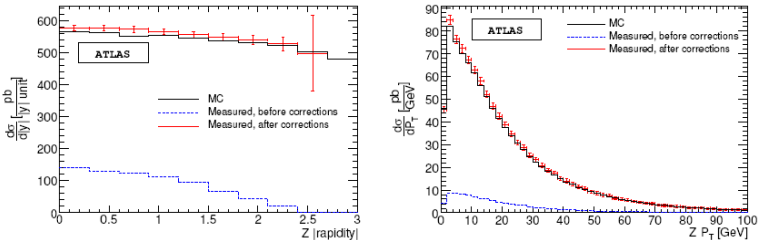
Рис. 11.9. Ожидаемые дифференциальные распределения Z -бозонов по быстроте (слева) и поперечному импульсу, соответствующие интегральной светимости 200 \text{ пб}^{-1} . Сплошной линией показаны MC события, пунктиром измеренные, точки с погрешностями соответствуют измерениям после введения необходимых поправок.
