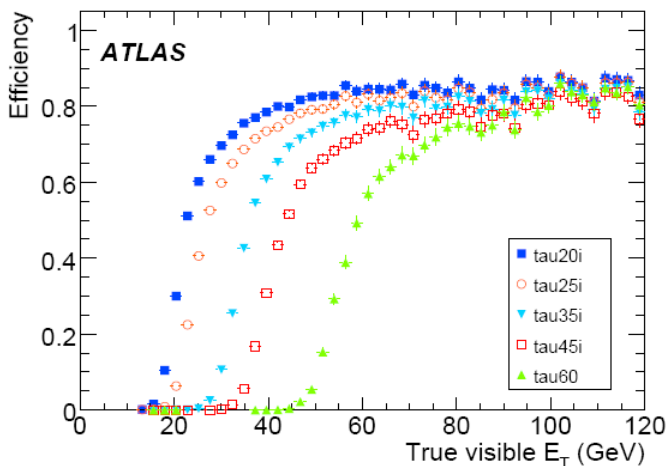
Рис.9.2. Суммарные эффективности триггера (L1+L2+фильтр событий) для отбора одиночного \tau -лептона при разных порогах триггера в детекторе ATLAS при начальной светимости.
