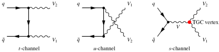
Рис.11.10. Фейнмановские диаграммы древесного уровня образования пар векторных бозонов на адронных коллайдерах. V, V1, V2 = \{W, Z, \gamma\} . В s-канале присутствует вершина связи трех бозонов TGC.
