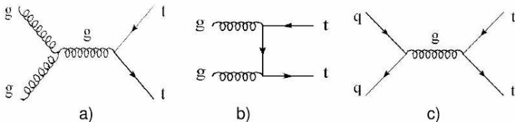
Рис.12.1. Диаграммы образования t -кварков в лидирующем порядке КХД : глюон-глюонное рассеяние (а), (b), кварк-кварковое рассеяние (с).
