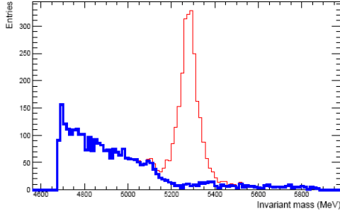
Рис.13.9. Распределение эффективных масс J/\psi K^+ для сигнальных событий распада V^+ -мезона (центральный пик) и комбинаторного фона от процессов bb \rightarrow \mu b \mu 4X . Поперечные импульсы мюонов > 6 ГэВ/с для первого и > 4 ГэВ/с для второго. Расстояние от точки рождения до точки распада \lambda > 0,1 мм
