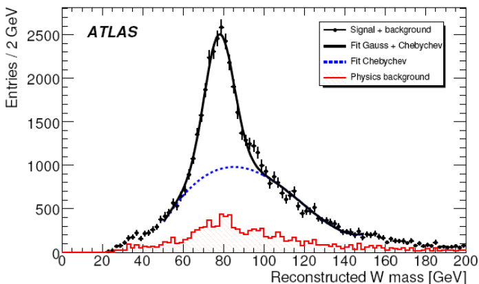
Рис.12.5. Инвариантная масса двух струй, которые отнесены к адронному распаду W . Сигнал и фон соответствуют интегральной светимости 1 \text{ fb}^{-1} . Для реконструкции струй использовался инклюзивный k_T -алгоритм в E схеме с радиусом струи R=0,4 . Точки соответствуют сигналу с фоном, нижняя гистограмма относится к фоновым событиям.
