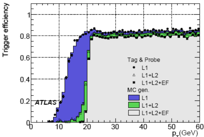
Рис.9.6. Сравнение эффективностей триггеров при регистрации мюонов в области больших поперечных импульсов при пороге 20 ГэВ/с, определенных моделированием МС и при использовании метода “tag and probe”.
