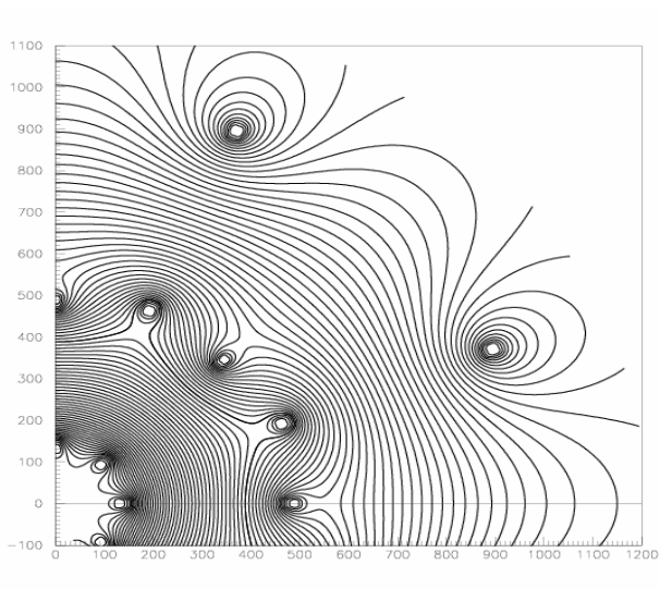
Рис.2.3. Силовые линии магнитного поля тороидальных магнитов детектора ATLAS в плоскости, перпендикулярной оси пучка. Размеры по осям приведены в мм. Частицы, вылетающие из точки соударения пучков (0,0) в поперечном направлении к оси пучка, испытывают максимальное воздействие на траекторию своего движения.
