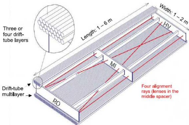
Рис.5.3. Схема камеры MDT.
