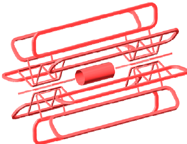
Рис.2.1. Схема элементов магнитной системы детектора ATLAS.
