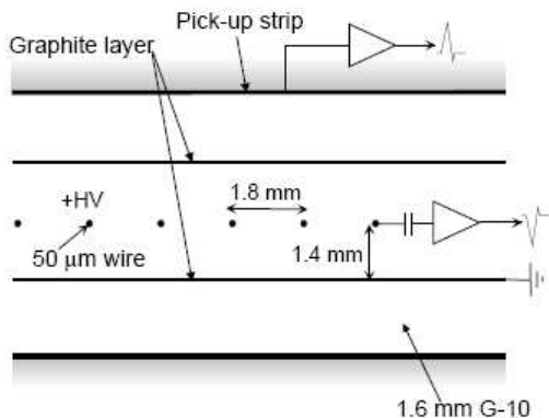
Рис.5.10. Схема камеры TGC. Показаны анодные проволоки, графитовые катоды, слой G-10 и катодные стрипы, направленные перпендикулярно проволокам. Диаметр проволоки 50 мкм.
