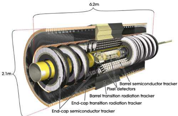
Рис.3.1 Схема Внутреннего детектора ATLAS. Показаны цилиндры и диски пиксельных детекторов (pixel detectors), цилиндры барреля и торцевые (End-cap) диски микростриповых кремниевых детекторов полупроводниковой трековой системы (semiconductor tracker, SCT) и внешний объем, занимаемый трековой системой переходного излучения (transition radiation tracker, TRT).
