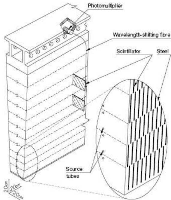
Рис.4.5. Схема сектора центрального блока тайл-калориметра детектора ATLAS.
