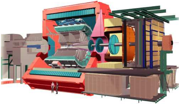
Рис.3. Общий вид детектора ALICE.
