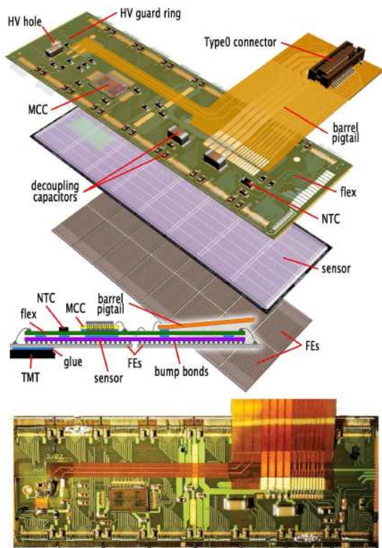
Рис.3.7. Фотография и схематическое изображение модуля пиксельных детекторов барреля. Дополнительные к приведенным
