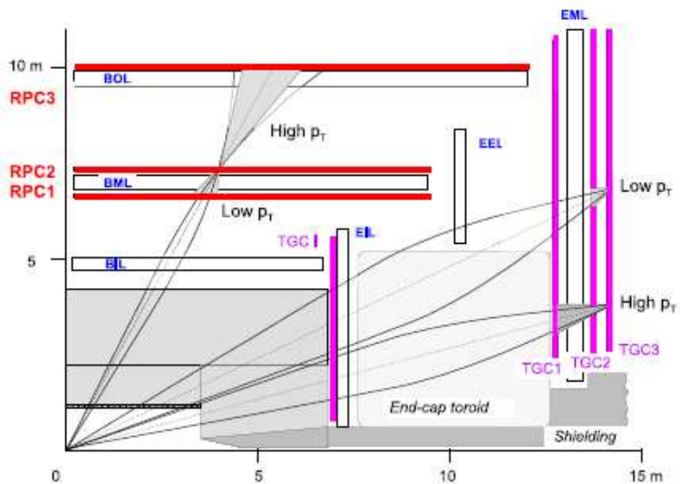
Рис.5.8. Схема размещения триггерных камер мюонного спектрометра ATLAS.
