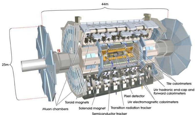
Рис.1.1. Схема детектора ATLAS. На схеме для удобства изображения отсутствуют две секции центрального тороида, половина больших торцевых дисков мюонных камер, сектор калориметров и внешней части Внутреннего детектора. Общая длина детектора 44 м, диаметр 25 м, вес 7000 т.
