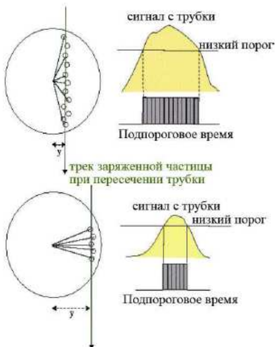
Рис.3.11. Схема прохождения заряженной частицы через трубку. Расстояние y координаты внутри трубки определяется по
