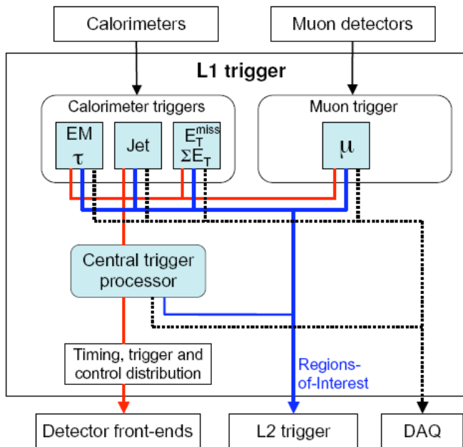
Рис.7.1. Блок-схема триггера первого уровня L1 детектора ATLAS. Решение принимает центральный процессор на основе данных калориметра и мюонного триггера. Показаны также линии связи с триггером второго уровня L2, формирующие области интересов RoI, и с системой сбора данных DAQ.
