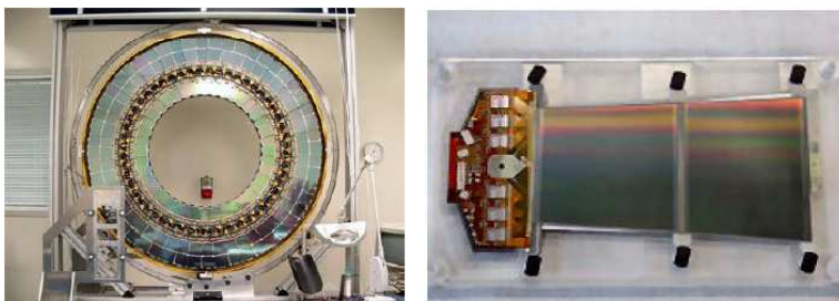
Рис.3.9. Фотографии диска SCT после сборки (слева) и одного из модулей диска модуля SCT (справа).
