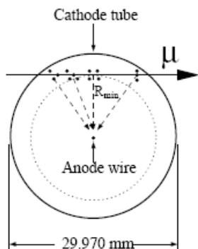
Рис.5.2. Сечение дрейфовой трубки камеры MDT.
