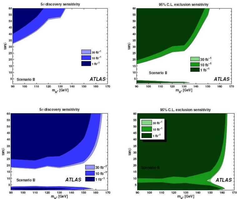
Рис.14.2.14. Ожидаемые результаты для канала t\tilde{t} \rightarrow bH+bW \rightarrow b\tau(ad\rho) vb lv (вверху) и канала t\tilde{t} \rightarrow bH+bW \rightarrow b\tau(ad\rho) vbqq (внизу). См. текст.
