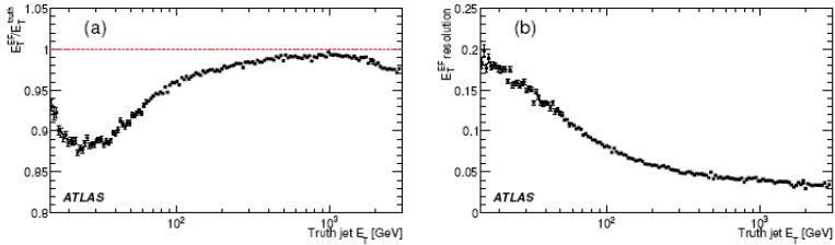
Рис.9.9. Энергетический масштаб поперечной энергии струй (а) и разрешение по энергии струй (б) в зависимости от истинной энергии струи E_T на уровне фильтра событий EF. Данные MC.
