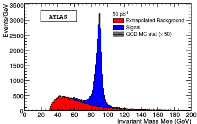
Рис.11.8. Реконструкция MC событий распада Z \rightarrow e\bar{e} на статистике 50 \text{ pb}^{-1} вместе с фоновыми событиями до введения ограничений по величину эффективной массы.
