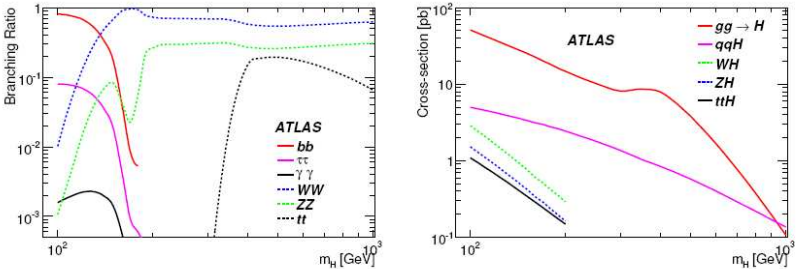
Рис.14.1.1а. Вероятности различных мод распада бозона Хиггса (слева) и сечений рождения бозона Хиггса в Стандартной модели для разных механизмов в пикобарнах в зависимости от массы бозона Хиггса.
