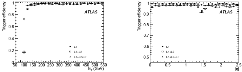
Рис.9.3. Эффективности триггеров разного уровня для электронов в зависимости от поперечной энергии электрона и псевдобыстроты для двух порогов триггера \epsilon 5 и \epsilon 105 .
