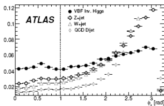
Рис.14.2.10. Переменная изолированности недостающей энергии I (слева) и разность азимутальных углов \phi_{jj} для сигнала невидимого бозона Хиггса с массой 130 ГэВ и трех типов фоновых событий. Распределения нормированы на единицу.
