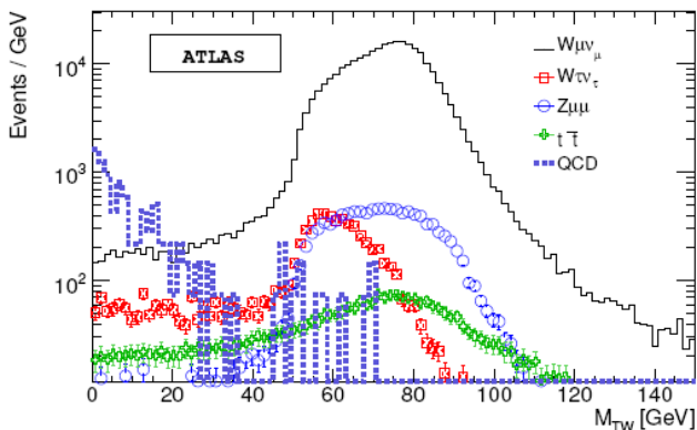
Рис.11.7. Реконструкция MC событий распада W \rightarrow \mu\nu на статистике 50 \text{ pb}^{-1} вместе с фоновыми событиями до введения ограничений на величину поперечной эффективной массы M_{T\bar{W}} .
