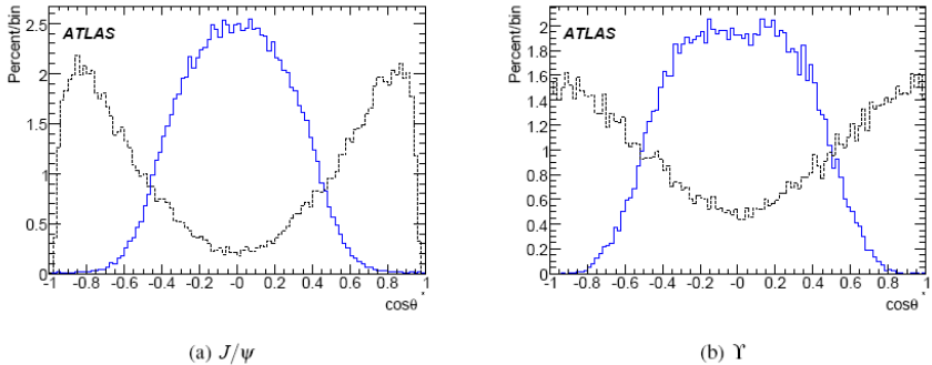
Рис. 13.4. Распределения реконструированных углов поляризации \cos \theta^* для J/\Psi и \Upsilon при пороге p_T мюонов 4\mu (сплошная гистограмма) и пороге 10\mu (штриховая гистограмма).
