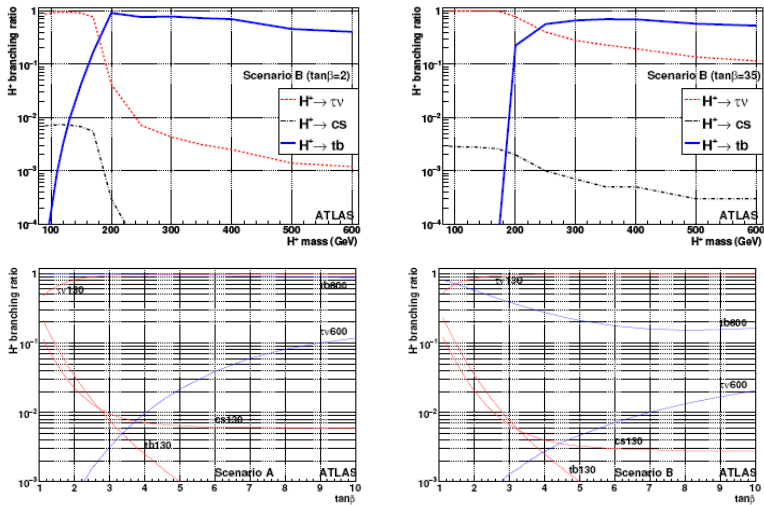
Рис.14.2.4. Рассчитанные вероятности различных каналов распада заряженного бозона Хиггса как функция его массы для сценария
