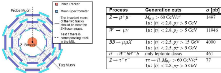
Рис.9.5. Иллюстрация метода “tag and probe” с использованием распадов Z \rightarrow \mu\mu для измерения эффективности триггера мюонов на данных эксперимента.
