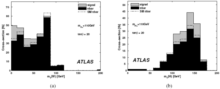
Рис.14.2.13. Распределения реконструированных поперечных масс H+ бозона для канал t\bar{t} \rightarrow bH + bW \rightarrow b\tau(adp) vbqq (вверху) и t\bar{t} \rightarrow bH + bW \rightarrow b\tau(lenm) vbqq (внизу) (См. текст).
