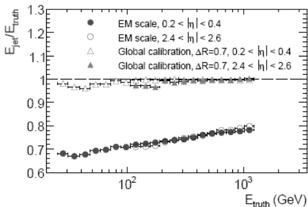
Рис.10.8.(а) Линейность расчетного отклика калориметра в зависимости от энергии струи E_{\text{truth}} .
