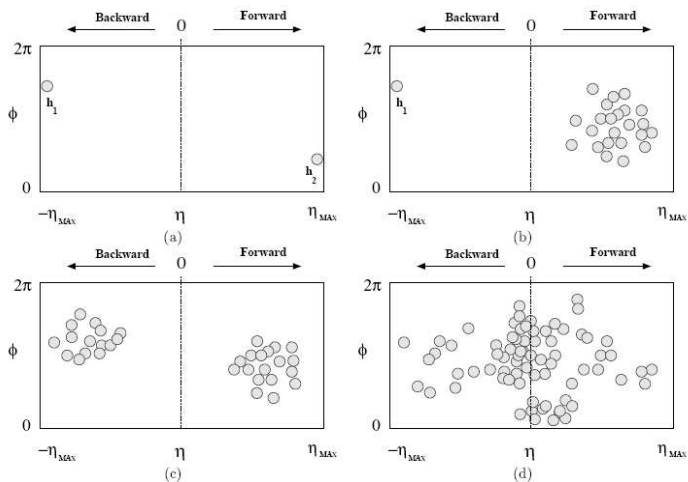
Рис.11.1. Расположение вторичных частиц при упругом взаимодействии протонов (а), в процессах одновершинной (b) и двухвершинной дифракции (с) и неупругом взаимодействии (d) в переменных псевдобыстроты \eta и азимутального угла \phi .
