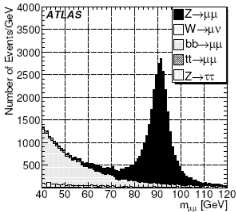
Рис.11.6. Реконструкция MC событий распада Z \rightarrow \mu\mu на статистике 50 \text{ пб}^{-1} вместе с фоновыми событиями до введения ограничений по величине эффективной массы и критерия изолированности.
