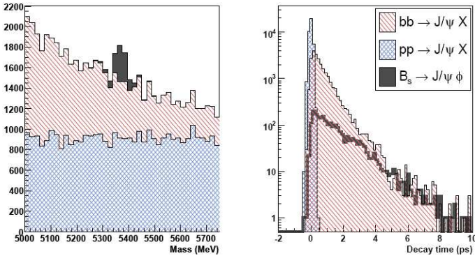
Рис.13.11. Распределения, аналогичные рисунку 13.10, для канала B_s^0 \rightarrow J/\psi\phi , где \phi \rightarrow K+K^- , J/\psi \rightarrow \mu\mu . Интегральная светимость распределений 150 \text{ пб}^{-1} .
