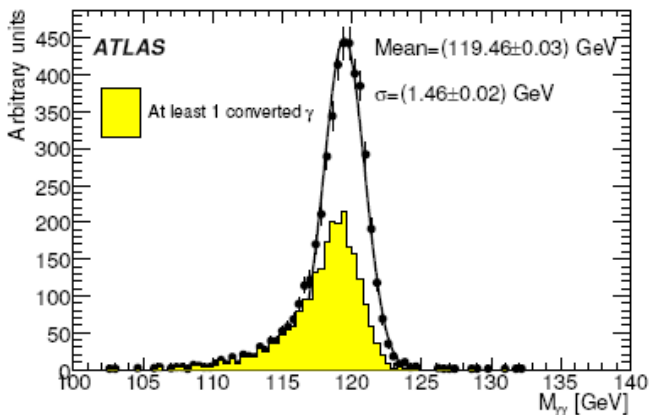
Рис.14.1.2 Распределение эффективных масс двух фотонов для распада бозона Хиггса с массой 120 ГэВ при учете дополнительного вещества в детекторе. Темная область соответствует вкладу фотонов с конверсией в детекторе.
