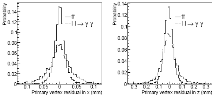
Рис.10.4. Разрешение восстановление координат точки соударения протонов в событиях с рождением пары топ-кварков и бозона Хиггса, распадающегося на два фотона: по переменной
