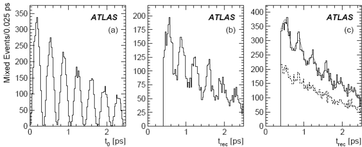
Рис. 13.20. Распределение B^0 s смешиваемых состояний с параметром \Delta m_s = 17,77 \text{ пс}^{-1} (a), то же распределение при учете конечного разрешения при измерении собственного времени жизни (b) и фоновых и неверно меченых событий (c). Пунктир – вклад фоновых событий без смешивания.
