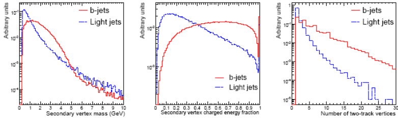
Рис.10.13. Эффективная масса частиц из вторичной вершины в струе (справа), доля энергии струи, уносимая этими частицами, и количество двух частичных вершин в струе (слева). Сплошные линии соответствуют струям b-кварков, пунктирные – струям от легких кварков.
