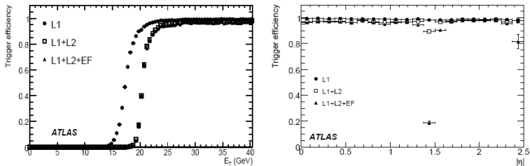
Рис.9.4. Эффективности триггеров разного уровня для фотонов в зависимости от поперечной энергии и псевдобыстроты для триггера g5 .
