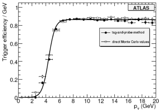
Рис.13.2. Эффективность триггера L1 регистрации мюонов с низкими поперечными импульсами. Темные точки получены методом tag-and-probe, светлые соответствуют MC расчетам эффективности.
