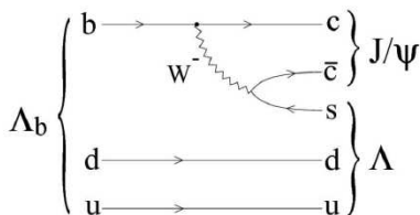
Рис.13.12. Диаграмма слабого распада \Lambda_b \rightarrow J/\psi \Lambda .
