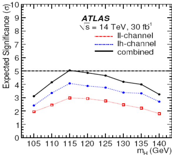
Рис.14.1.10. Значимость сигнала распада H \rightarrow \tau^+ \tau^- , ожидаемая для нескольких значений массы бозона Хиггса при интегральной светимости 30 \text{ fb}^{-1} для типов распада \tau -лептонов ( lh ) и ( ll ).
