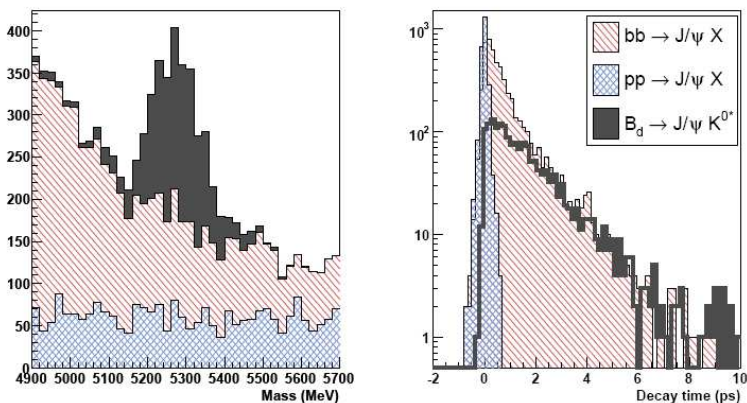
Рис.13.10. Распределение реконструированных масс B_d^0 (слева) и собственного времени жизни B-мезонов в распаде B_d^0 \rightarrow J/\Psi K^{0*} при интегральной светимости 10 \text{ пб}^{-1} для моделированных событий сигнала (темная область) и фоновых событий pp \rightarrow J/\Psi X и bb \rightarrow J/\Psi X .
