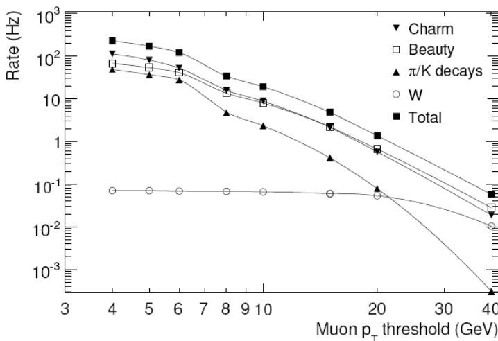
Рис.8.3. Скорости потоков мюонов в зависимости от величины порога p_T при светимости 10^{31} \text{ см}^{-2} \text{ с}^{-1} и для различных процессов генерации. Темными квадратами отмечен суммарный спектр.
