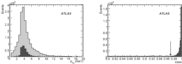
Рис.13.8. Распределения по p_T фотонов в событиях с рождением J/\Psi (слева) и по \cos \alpha угла вылета фотонов относительно направления J/\Psi (справа). Пояснения см. текст.
