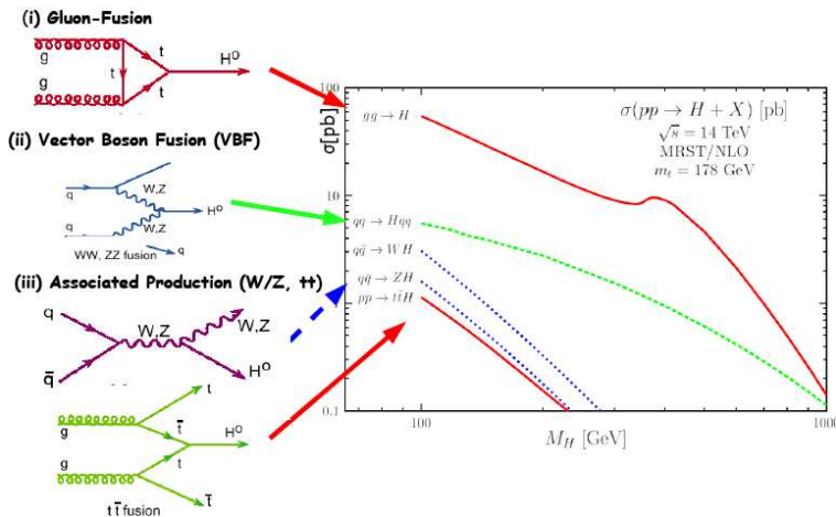
Рис.14.1.16. Диаграммы, соответствующие различным механизмам образования H-бозона на рис.14.1.1а: (i)слияния глюонов, (ii) слияние векторных бозонов (VBF), (iii) ассоциированное рождение (в сопровождении W, Z или tt). (C.Weiser, ATL-PHYS-SLIDE-2009-234).
