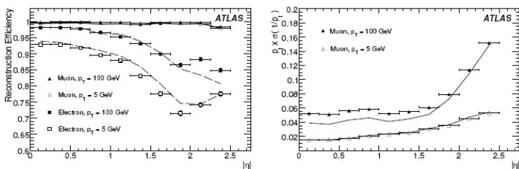
Рис.9.1. Эффективности реконструкции (слева) и разрешение при определении импульсов треков электронов и мюонов в зависимости от псевдобыстроты трека |\eta| .
