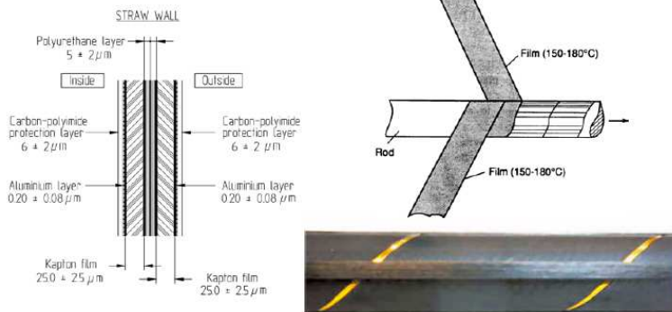
Рис.3.10. Структура стенки трубки Детектора переходного излучения (слева), процесс изготовления трубки (справа сверху) и фотография готовой трубки с приклеенной вдоль оси трубки нити углепластика.
