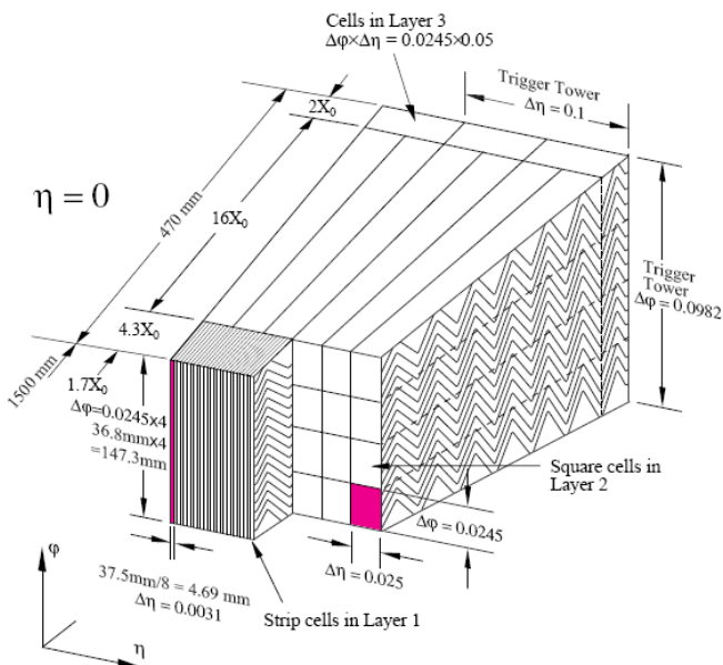
Рис.4.3. Рисунок модуля барреля EM калориметра. Видны его три слоя и расходимость электродов по азимутальному углу \varphi . Вес половины барреля 57 т.
