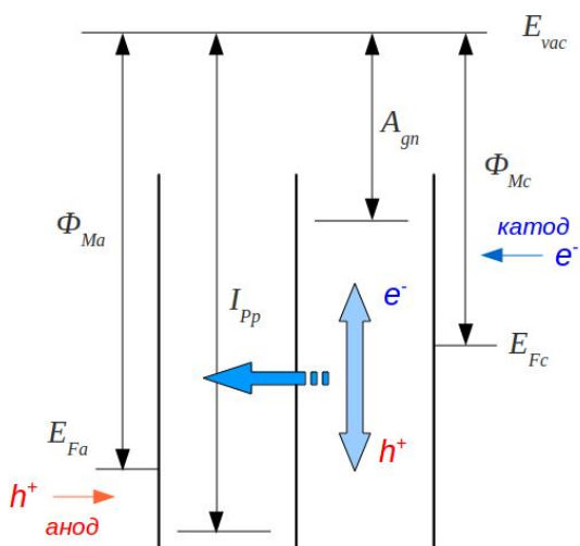
Рис. 3. Энергетическая диаграмма органического светодиода
