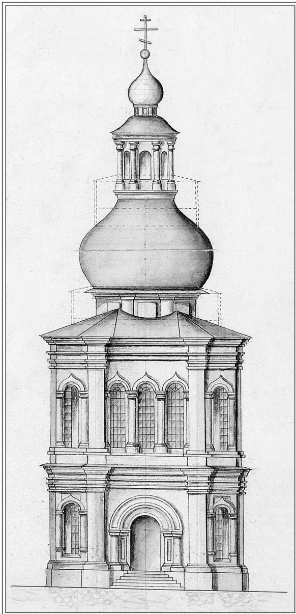
Проект переделки церкви на Секирной горе для устройства на ней маяка. 1861 г. РГА ВМФ. Ф. 402. Оп. 2. Д. 1101. Л. 10.
