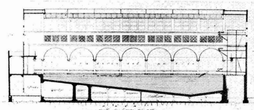
Sección longitudinal de la sala de la piscina
