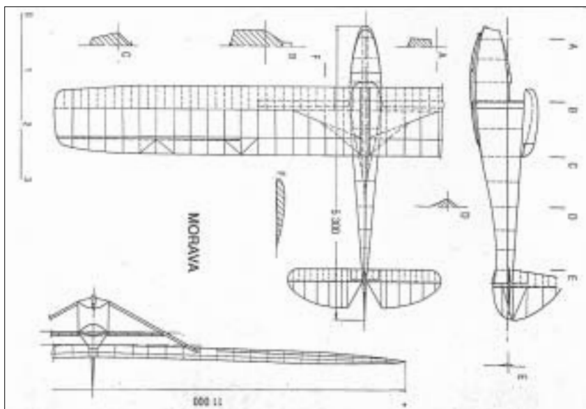
Větroň „Morava“. Konstruktor Jan Hrbek, rok vzniku 1933
