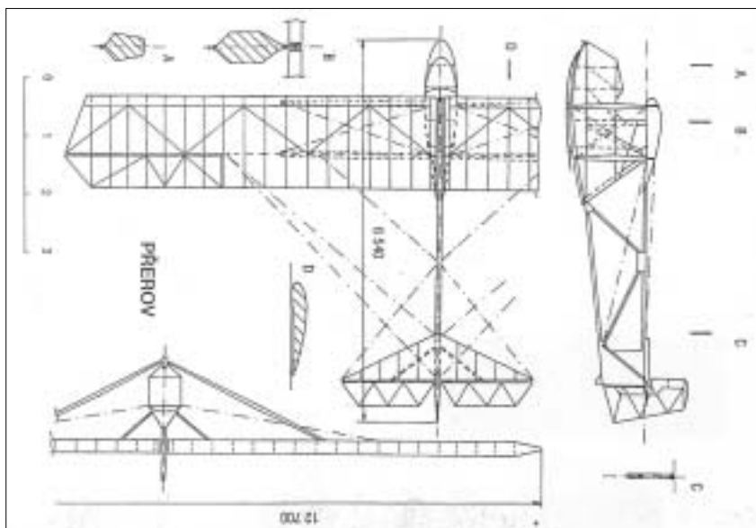
Kluzák „Přerov“. Konstruktor Jan Hrbek, rok vzniku 1933
