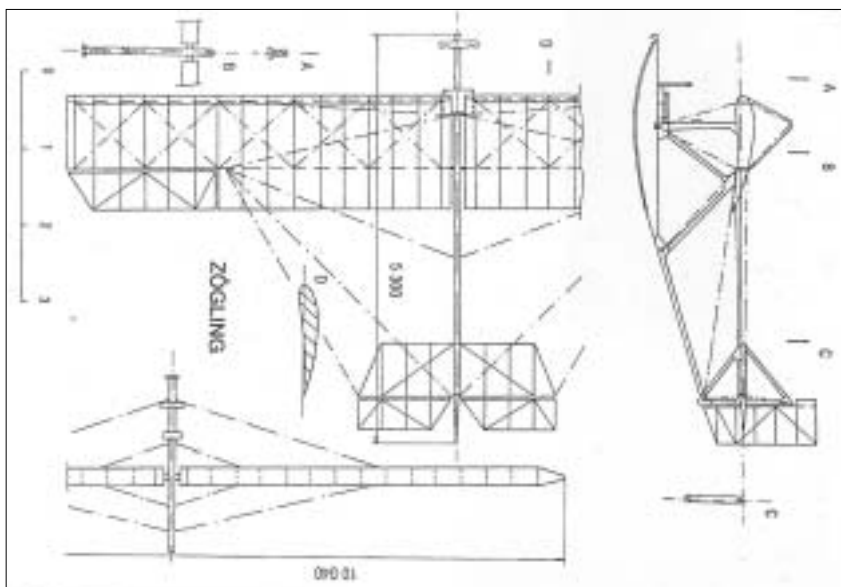
Kluzák „Zögling“. Konstruktéři Fritz Stamer, Alexander Lippisch, rok vzniku 1930, Německo
