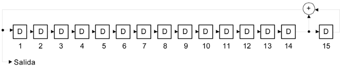
Figura 10 — Generación del polinomio PRBS y circuito
