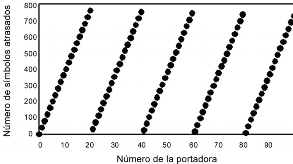
Figura 26 — Arreglo de las portadoras siguiendo el entrelazamiento temporal (modo 1, l = 8)
