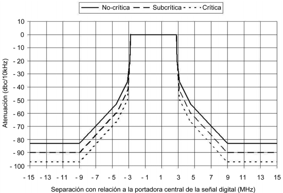
Figura 38 — Máscara del espectro de transmisión para radiodifusión de televisión digital terrestre
