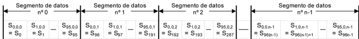
Arreglo de símbolos antes del interleaving
