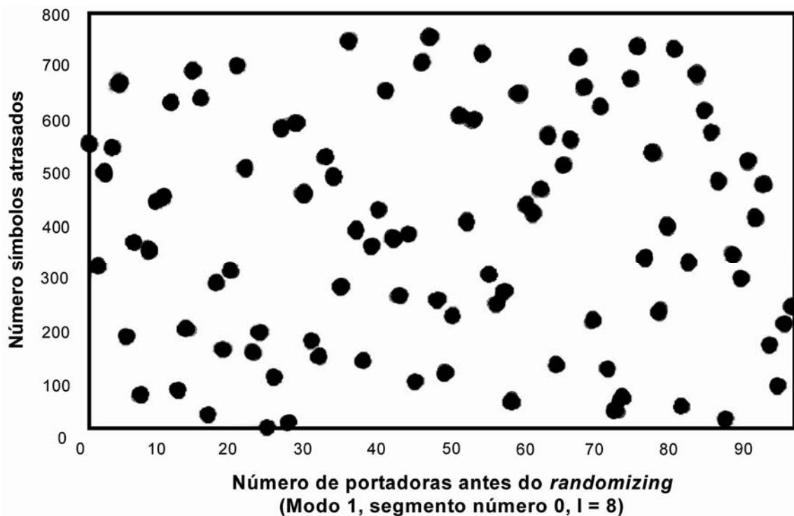
Figura 31 — Ejemplo de arreglo de las portadoras después del entrelazamiento en tiempo y de la randomizing de las portadoras
