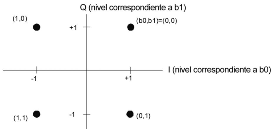
Figura 17 — Constelación QPSK
