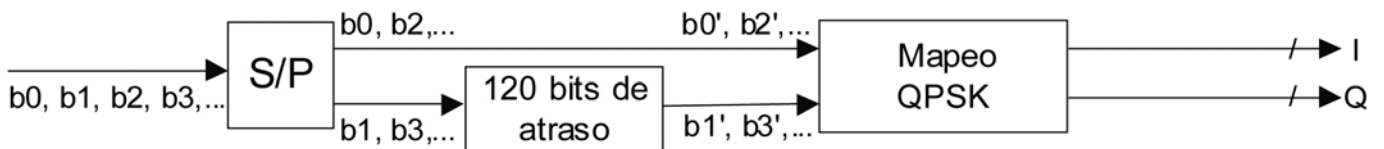
Figura 16 — Diagrama del sistema de modulación QPSK
