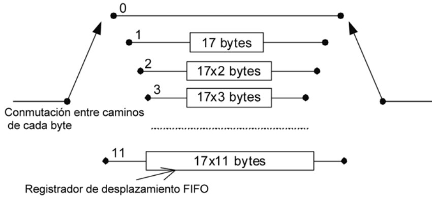
Figura 11 — Circuito de byte interleaving
