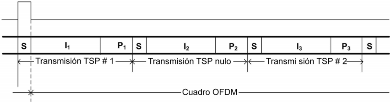
Sincronismo de cuadro OFDM
