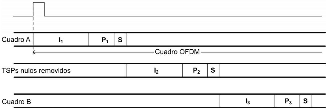
Figura 9 — Ejemplo de división del TS en dos capas jerárquicas
