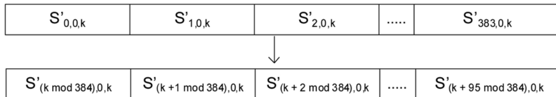
c) Rotación de portadora en el modo 3
