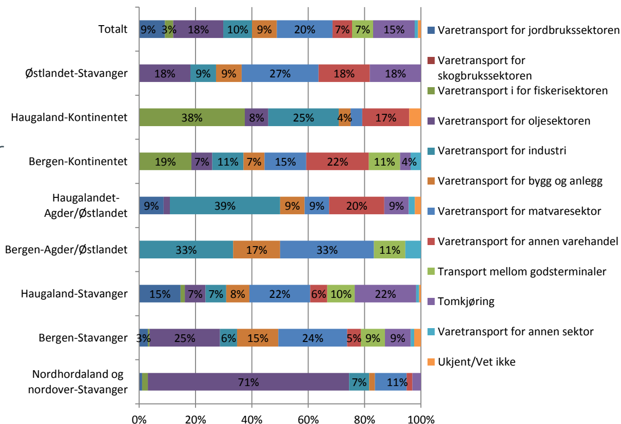
Figur 24 Fordeling av lastebilturner over Mortavika-Arsvågen etter sektor og transportkorridor.
