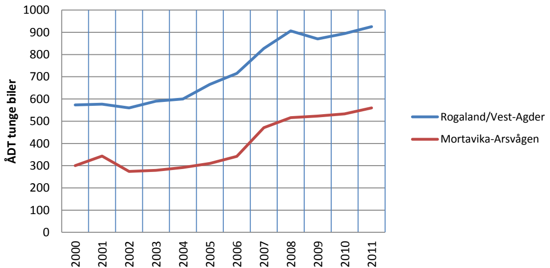
Figur 17 Utvikling i antall tunge kjøretøy ved Mortavika-Arsvågen, og ved Tronvik på grensen mellom Rogaland og Vest-Agder i perioden 2000-2011. Kilde: IRIS rapport 2010/061.
