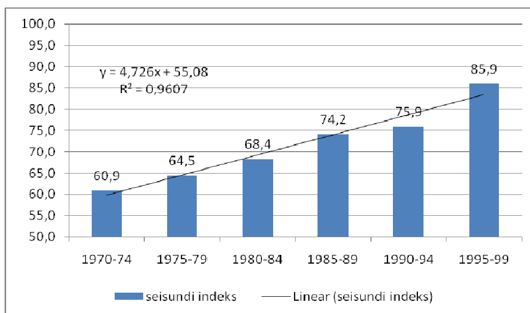
Graafik 13. 1970-1999 ehitatud sildade Seisundi Indeksid
