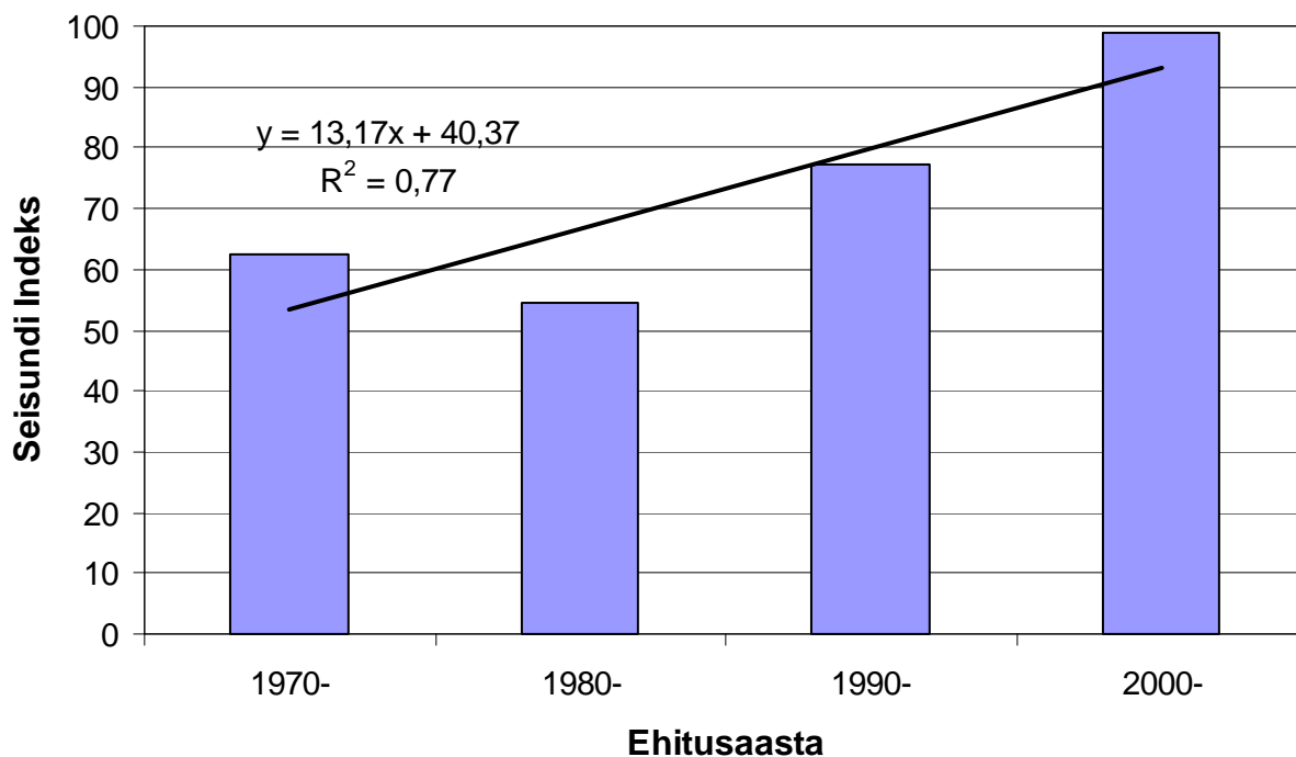
Erinevatel aastakümnetel ehitatud kaldasamba istepatjade SI-d
