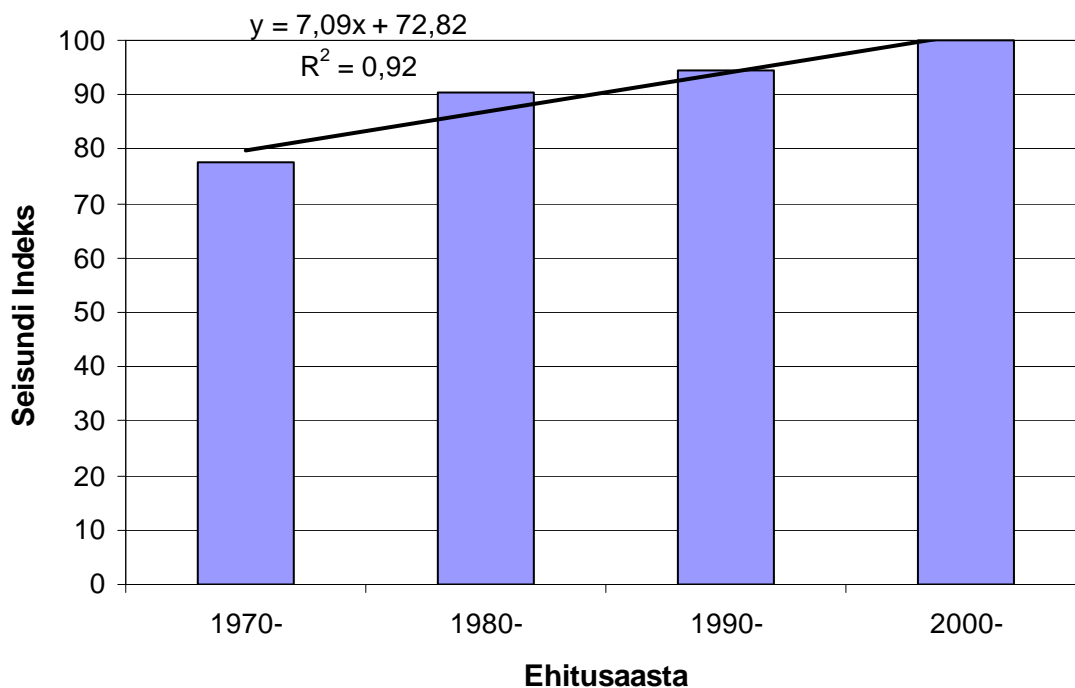
Erinevatel aastakümnetel ehitatud hüdroisolatsioonide SI-d
