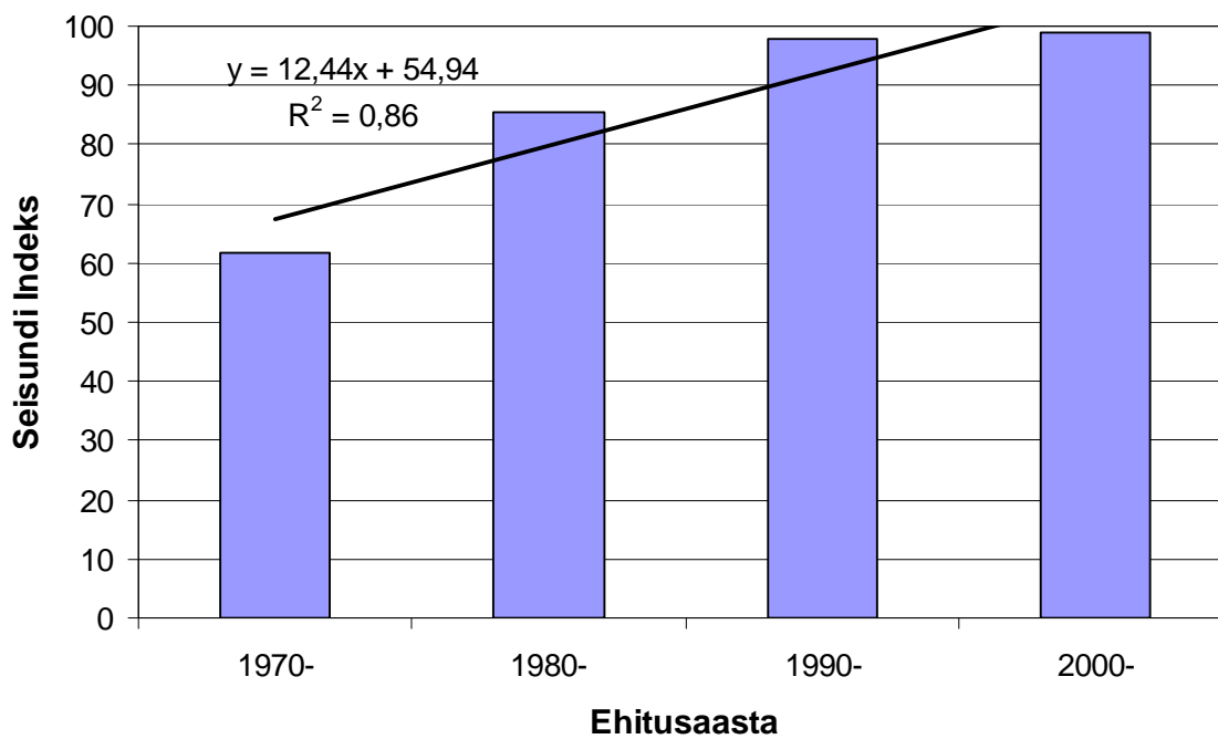
Erinevatel aastakümnetel ehitatud eelpingestatud talade SI-d
