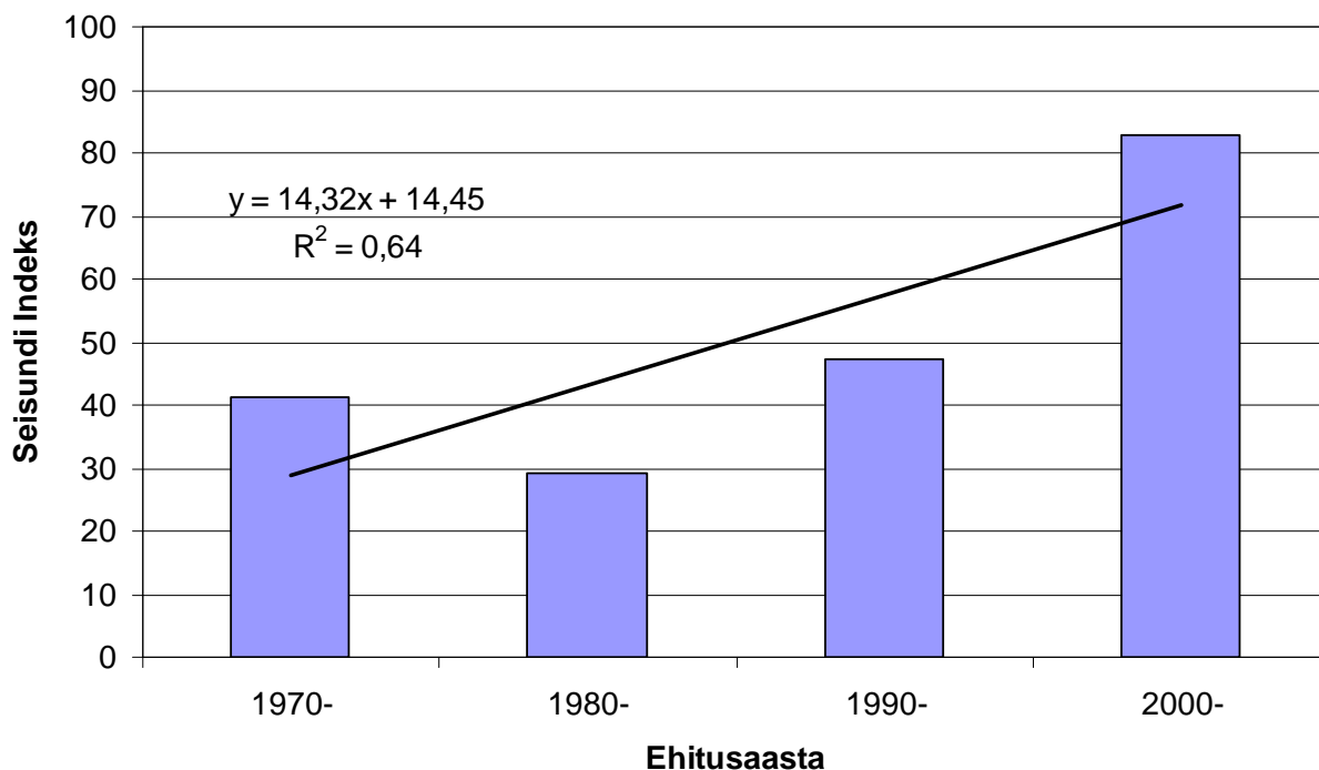
Erinevatel aastakümnetel ehitatud deformatsioonivuukide SI-d
