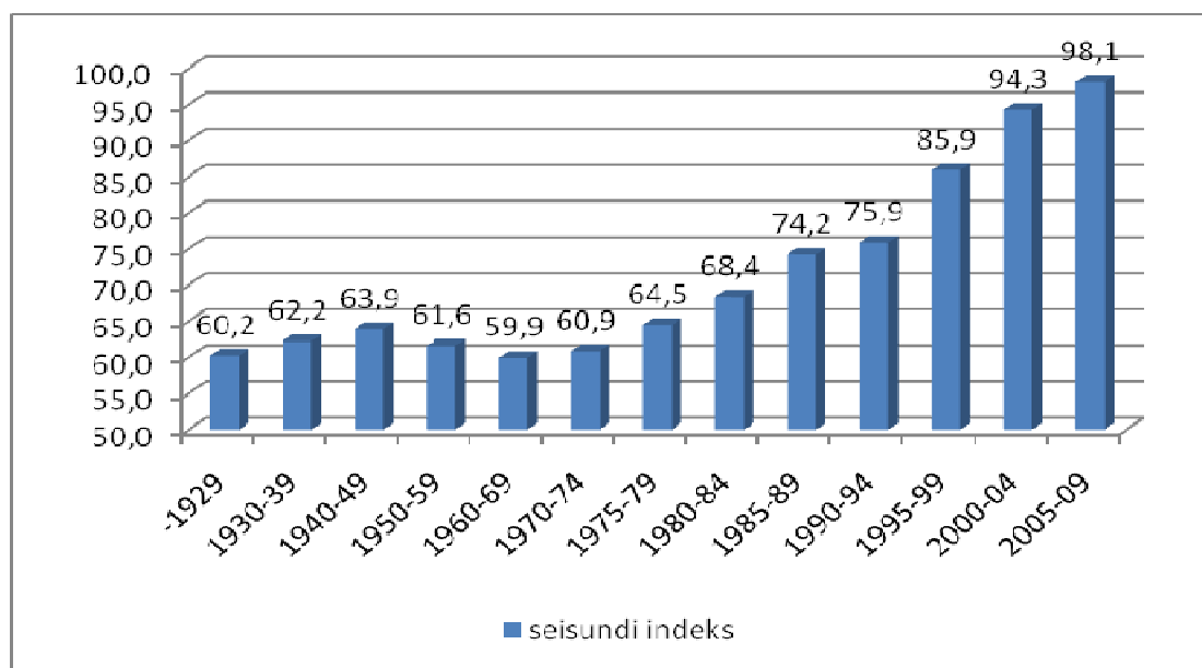
Graafik 8. Erinevatel aastakümnetel ehitatud sildade Seisundi Indeks, mis pole läbinud remonti
