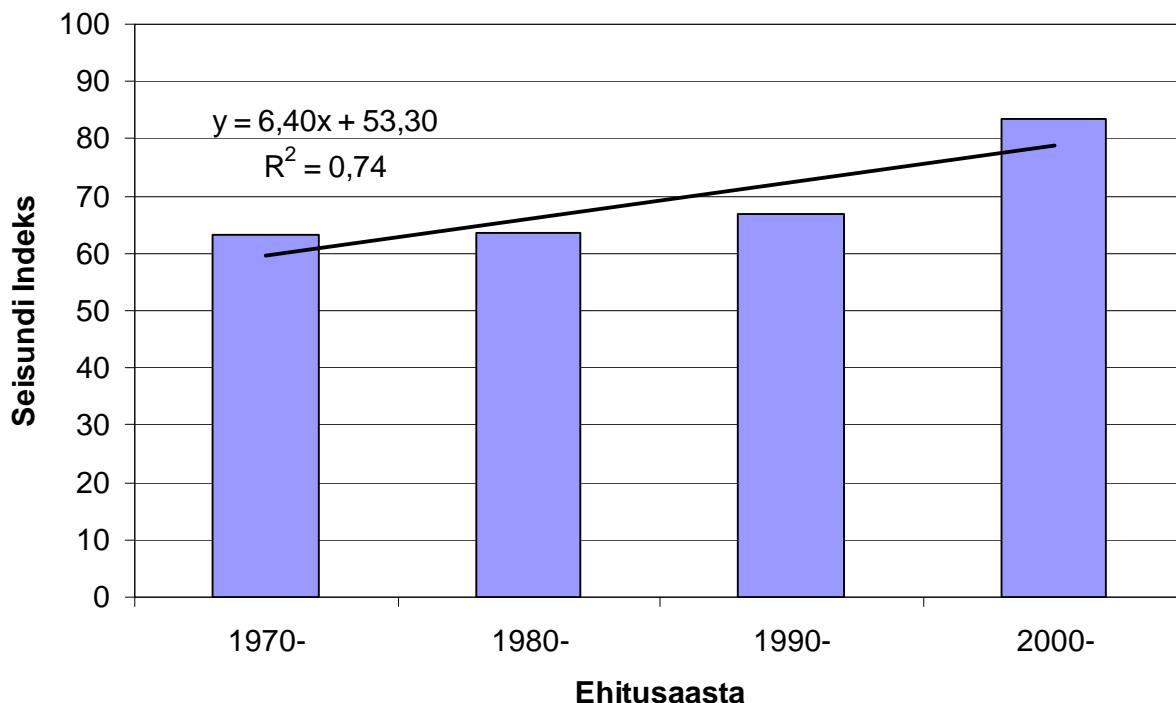
Erinevatel aastakümnetel ehitatud pealesõiduplaatide SI-d
