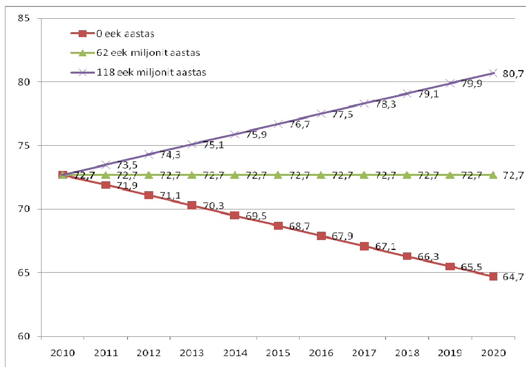
Graafik 14. Sillavõrgu Seisundi Indeksi muutus erinevate investeeringu strateegiatega korral
