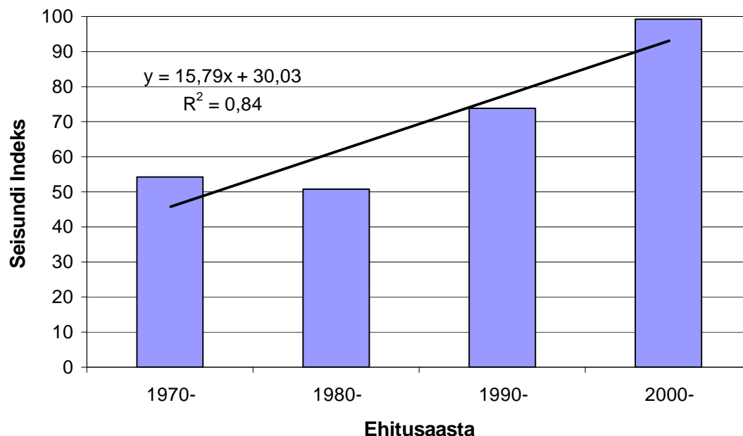
Erinevatel aastakümnetel ehitatud silla käsipuude SI-d
