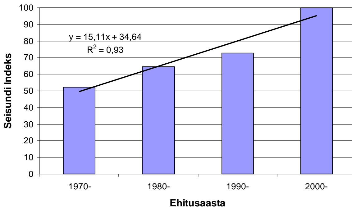
Erinevatel aastakümnetel ehitatud r/b vaiade SI-d
