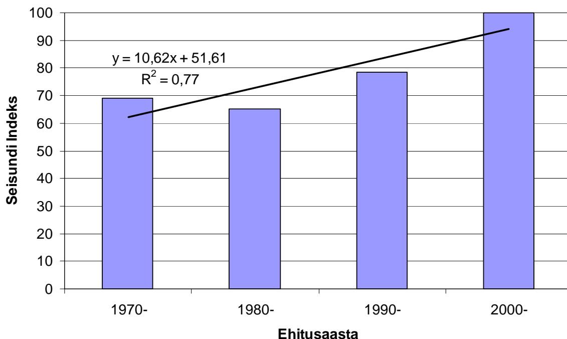
Erinevatel aastakümnetel ehitatud r/b postde SI-d
