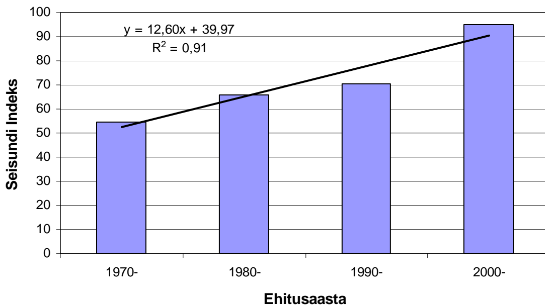
Erinevatel aastakümnetel ehitatud sõidutee katete SI-d
