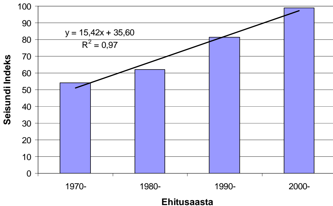
Erinevatel aastakümnetel ehitatud eelpingestatud talade SI-d
