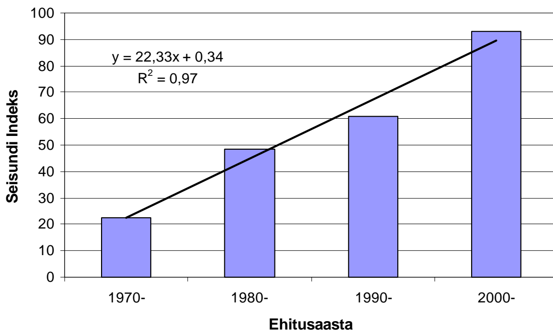
Erinevatel aastakümnetel ehitatud mahasõidu pörkepiirete SI-d
