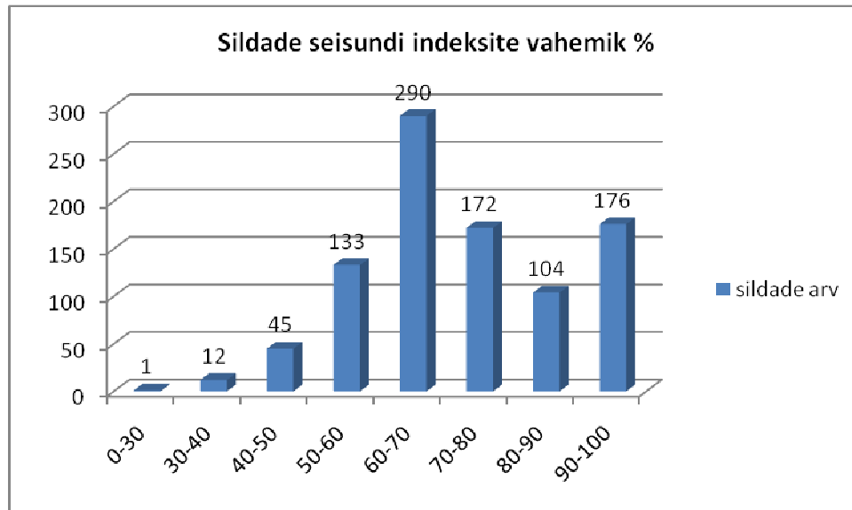
Graafik 7. Sildade jagunemine SI vahemike kaupa
