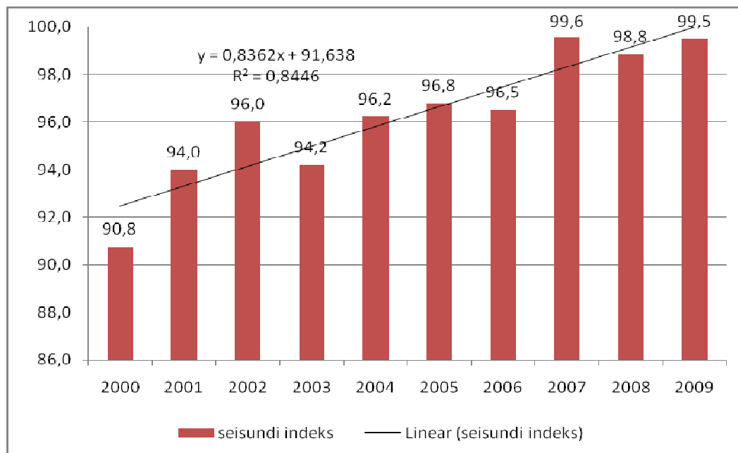
Graafik 12. Viimase 10 aasta jooksul ehitatud sildade SI-d 2010. aastal
