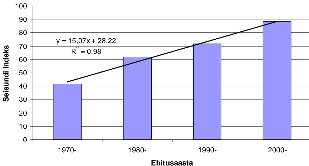
Erinevatel aastakümnetel ehitatud koonusekindlustuste SI-d
