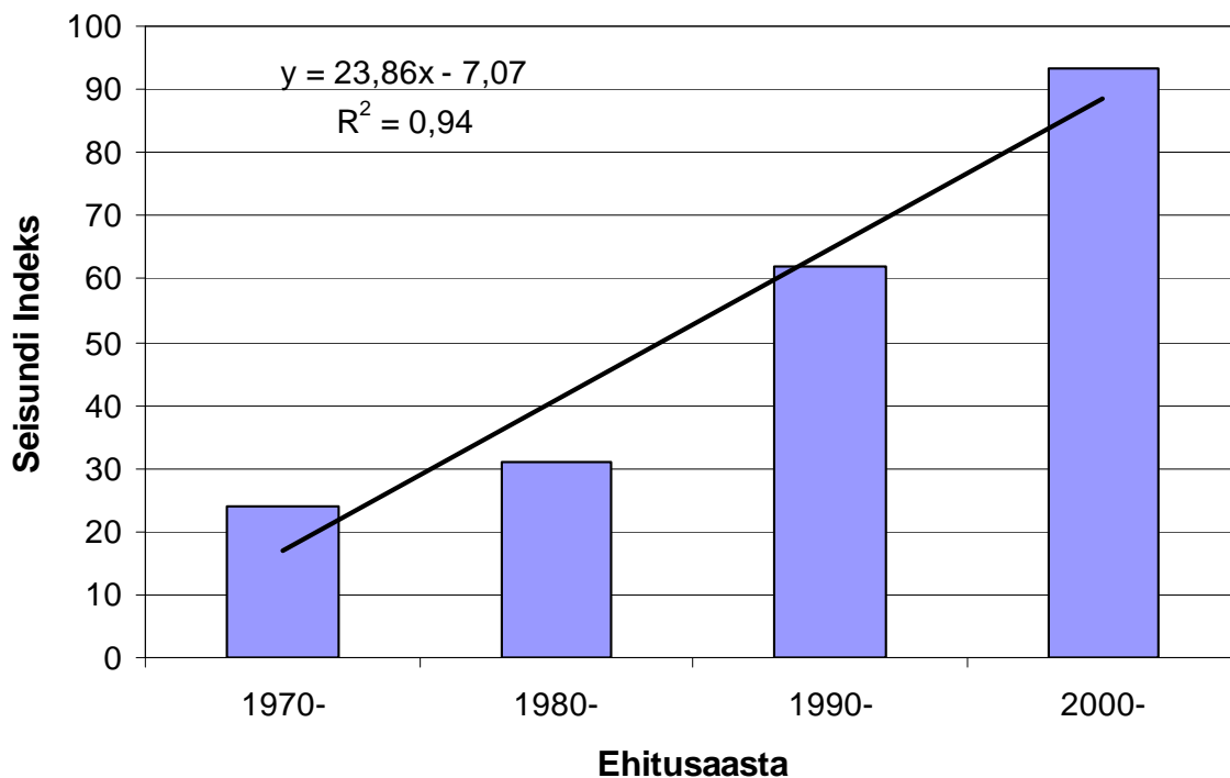
Erinevatel aastakümnetel ehitatud joatorude SI-d
