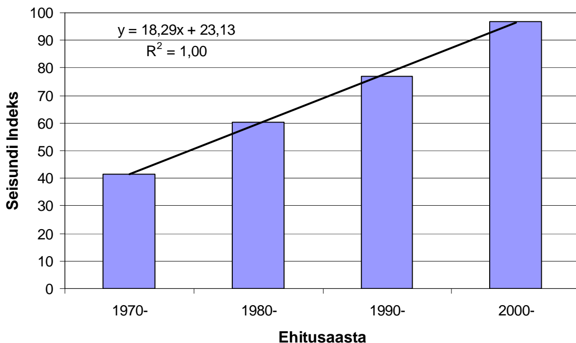
Erinevatel aastakümnetel ehitatud silla pörkepiirete SI-d
