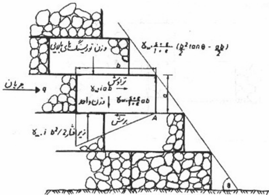
شکل شماره ۲۲ - سازه توریسنگی پلکانی و نیروهای وارده بر آن (جوان و همکاران ، ۱۳۷۹)
