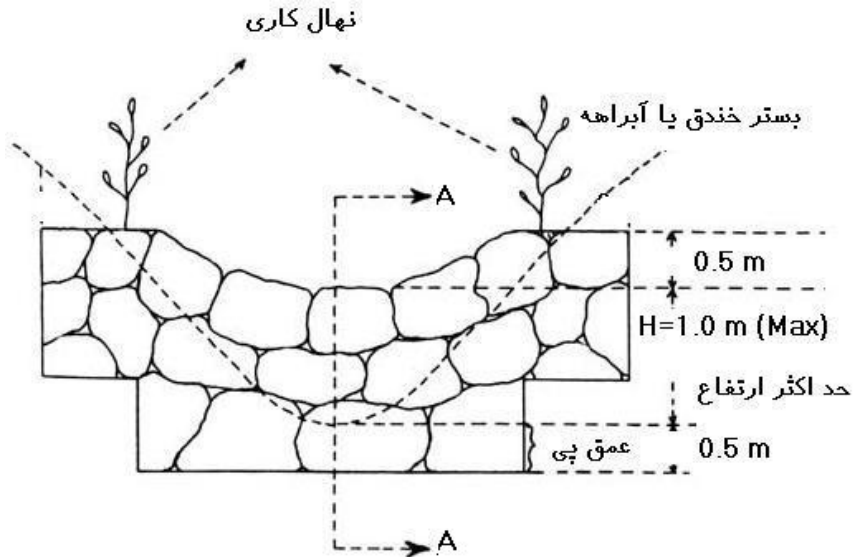
شکل شماره ۹- نمای جلوی بند اصلاحی خشک‌چین (Geyik ، ۱۹۸۶)
