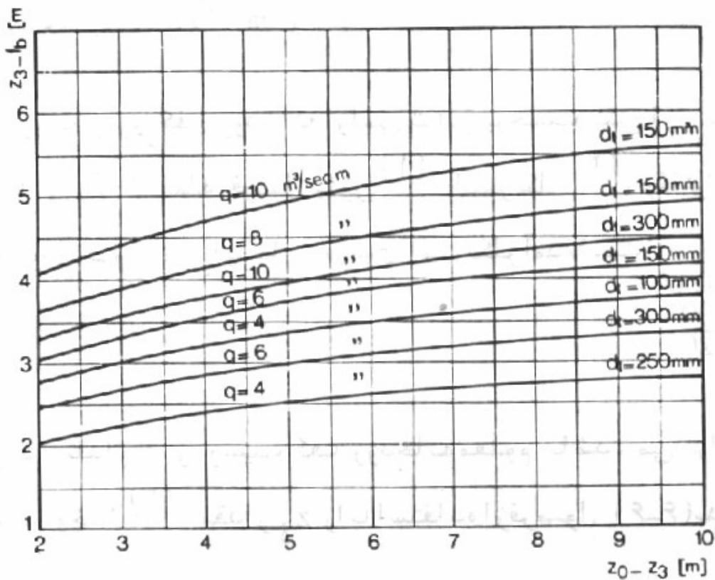
شکل ۳۳: تغییرات عمق آب شستگی بنا بر فرمول شوکلیتیج (جوان و همکاران، ۱۳۶۹)
