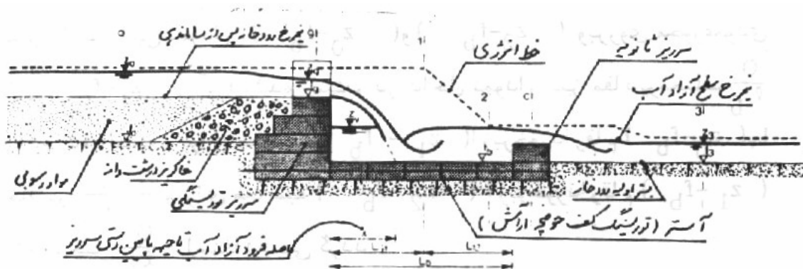
شکل ۳۵: رفتار هیدرولیکی سرریزی تا سطح تاج خاکریزی شده (جوان و همکاران، ۱۳۶۹)
