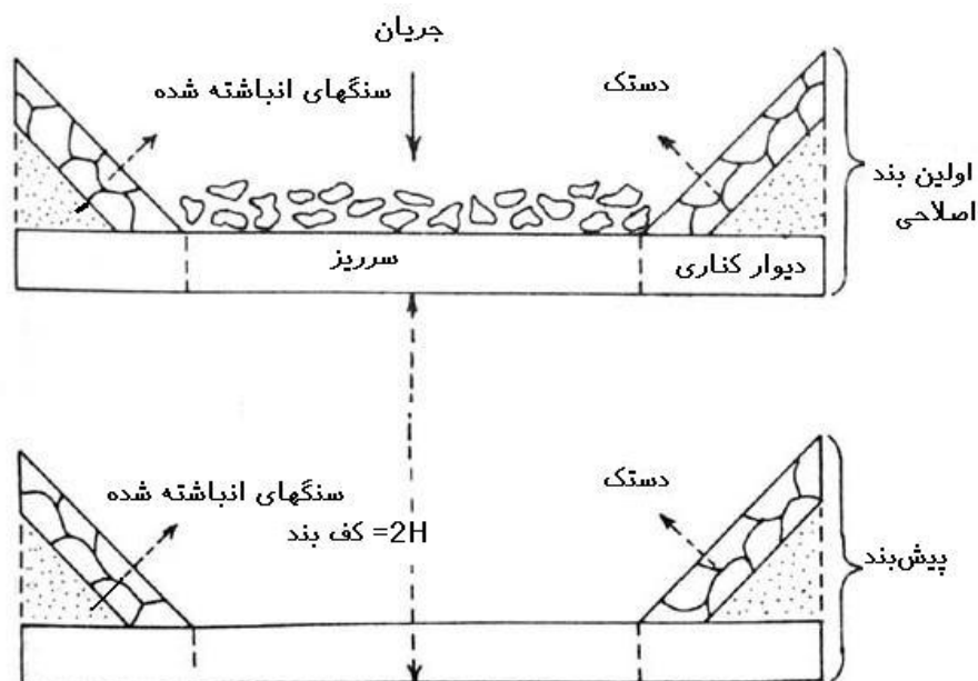
شکل شماره ۱۱- تصویر اولین بند اصلاحی خشکه چین همراه با پیش بند (Geyik ، ۱۹۸۶)
