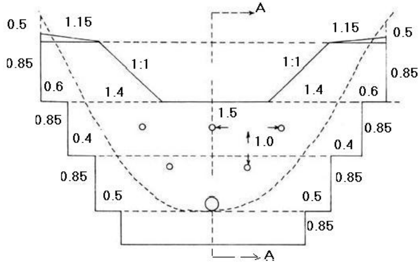
شکل شماره ۱۷ - نمای جلو اولین بند اصلاحی توریسنگی (Geyik، ۱۹۸۶)
