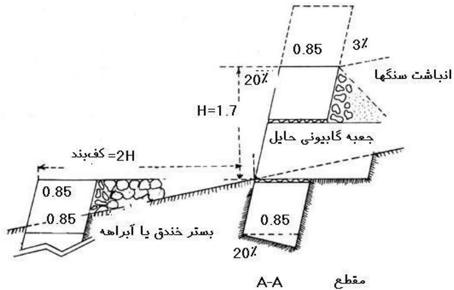
شکل شماره ۱۸ - مقطع اولین بند اصلاحی توریسنگی با پیش‌بند (Geyik، ۱۹۸۶)
