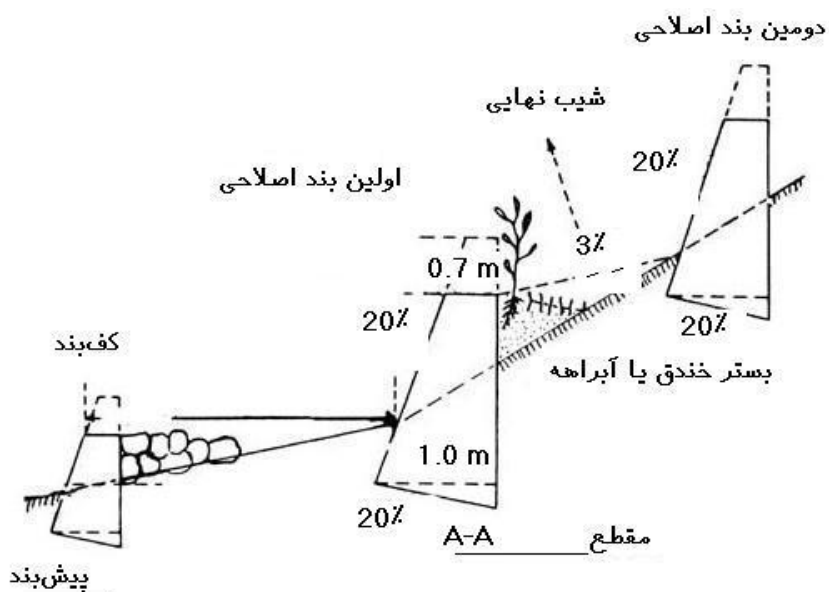
شکل شماره ۱۰- مقطع اولین بند اصلاحی خشکه چین همراه با پیش بند (Geyik ، ۱۹۸۶)
