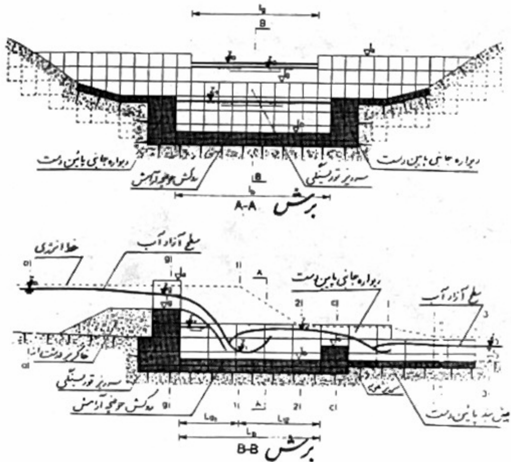
شکل ۲۸ - سرریز توریسنگی قائم با حوضچه آرامش آستردار همسطح با بستر رودخانه (جوان و همکاران، ۱۳۶۹)
