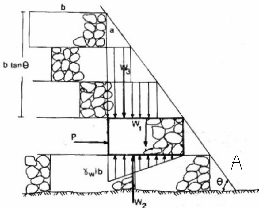
شکل شماره ۲۳- نیروهای وارده بر پیکر آزاد یک واحد توریسنگی در یک سازه پلکانی (جوان و همکاران ، ۱۳۷۹)
