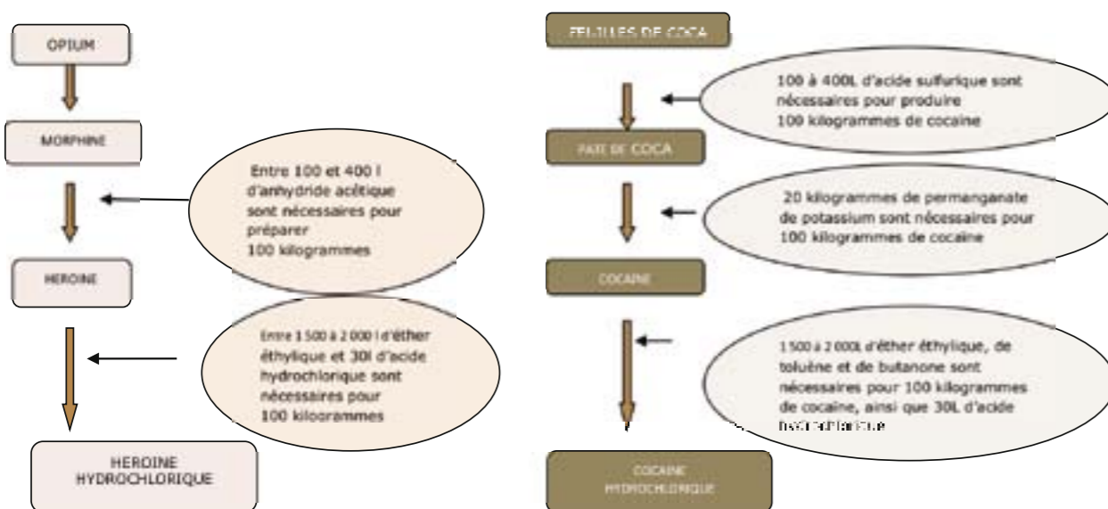
Schéma 1. L'usage des précurseurs dans la fabrication de la cocaïne et de l'héroïne.
