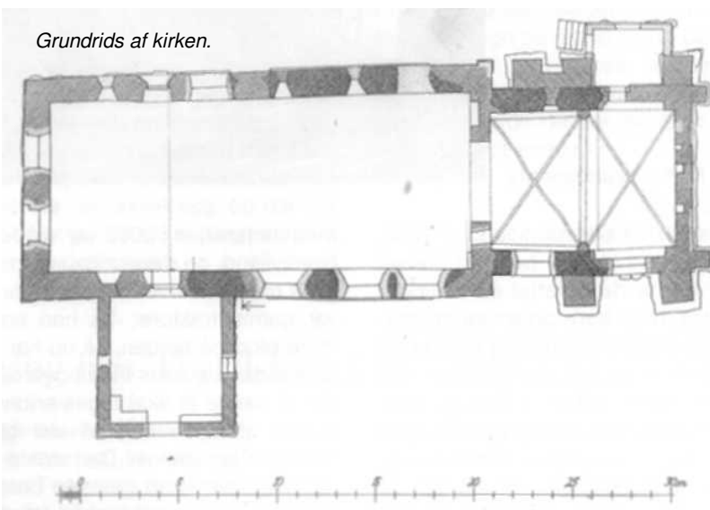
Hørup kirke Plan. 1:300. Målt af John Petersen 1957. Tegnet af Holger Schmidt 1961.
