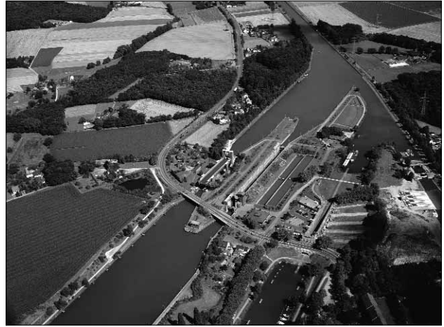
Neues Schiffshebewerk Henrichenburg in Waltrup, Recklinghausen, 1998 Fotograf: Stuttgarter Luftbild Elsässer
