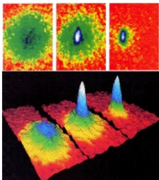
Fig.1. Prima observare experimentală a fenomenului CBE în rubidiu.
