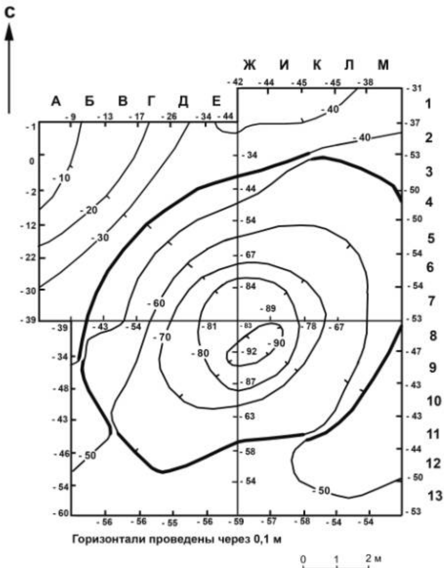
Рис. 2. Селище Заводоуковское 9. Нивелировочный план раскопа
