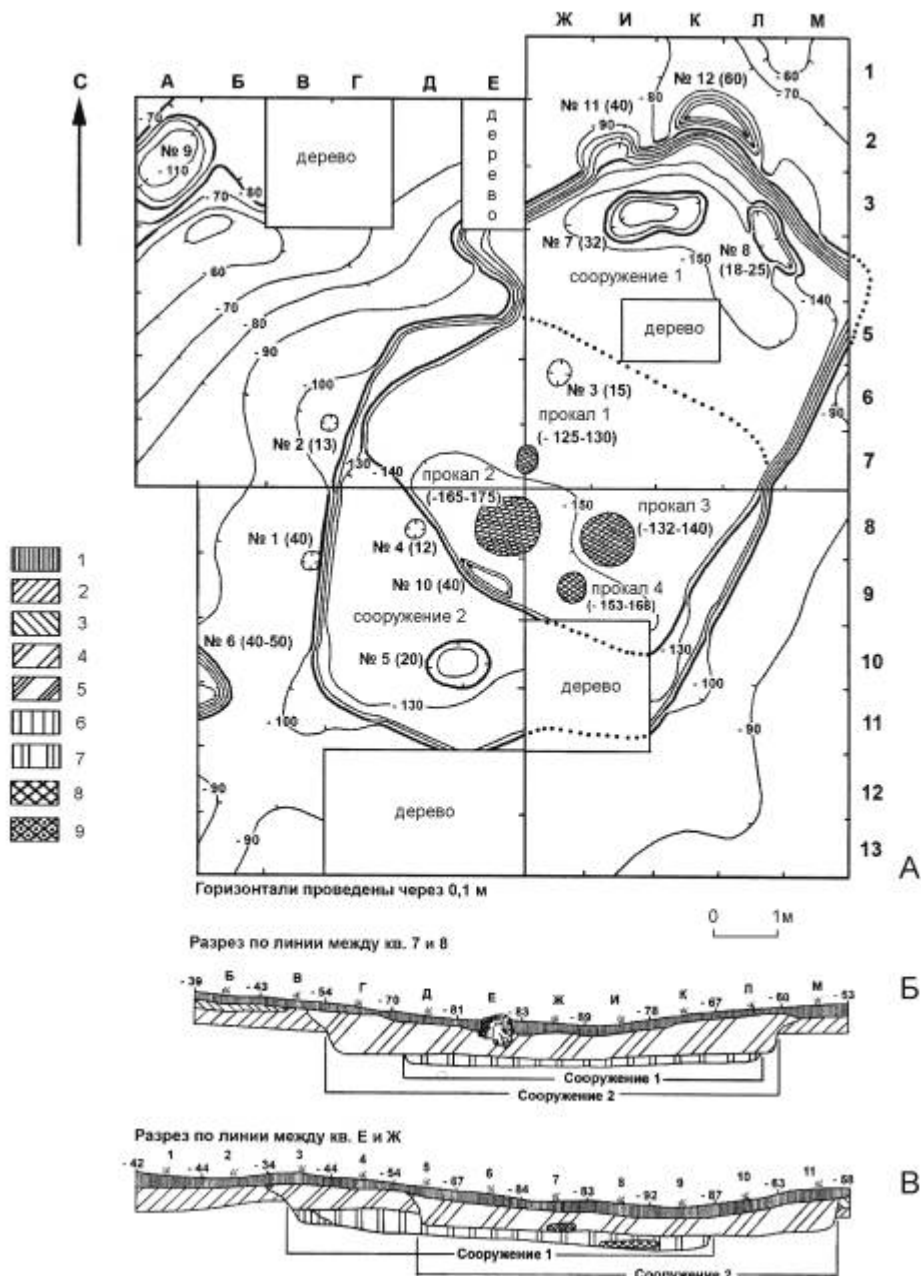
Рис. 3. Селище Заводоуковское 9. План (А) и разрезы (Б и В) раскопа: 1 — дерново-гумусный слой; 2 — светло-коричневая супесь; 3 — супесь горчичного цвета; 4 — коричневая супесь; 5 — темно-коричневая супесь; 6 — светло-серая супесь; 7 — серая супесь; 8 — прокал эпохи неолита; 9 — прокал бронзового века.
