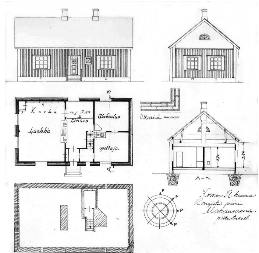
Ryppylänmäen koulun rakennuskuvia
