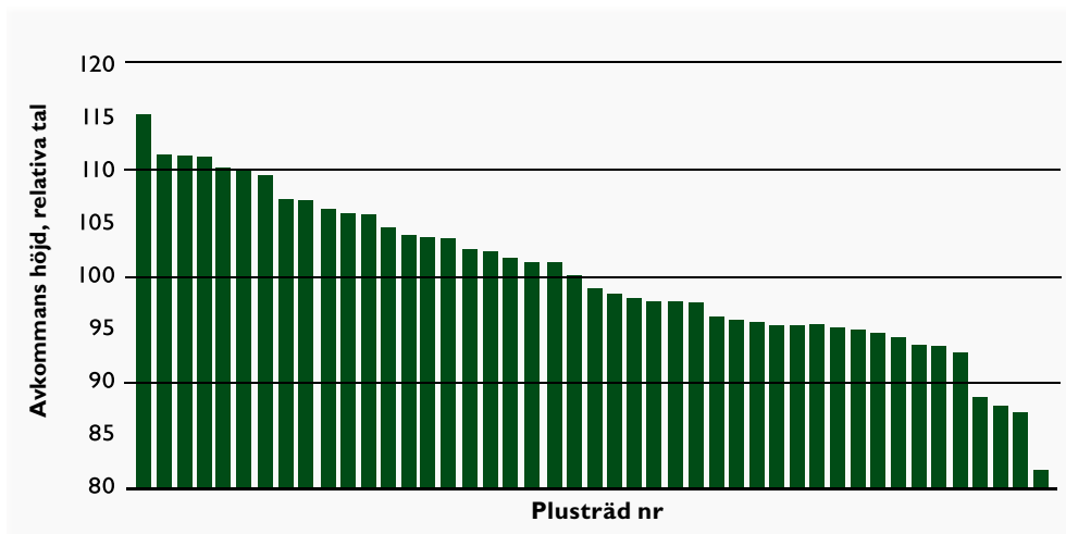
Figur PR8 Resultat av avelsvärdering av plusträd för tallförädlingspopulationen T15. 58
