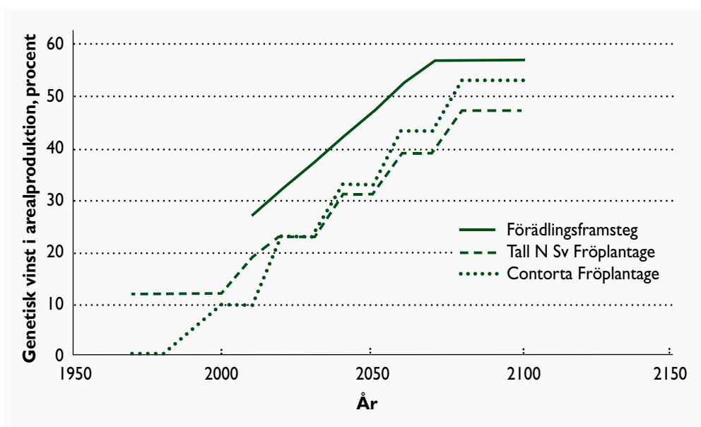
Figur PR5 Förädlingsvinster i arealproduktion, exemplifierade med tall och contortatall i norra Sverige, realiserade genom fröplantor från plantager eller från vegetativ förnygring (vinster utan avdrag för inväxning av vilda plantor). 52
