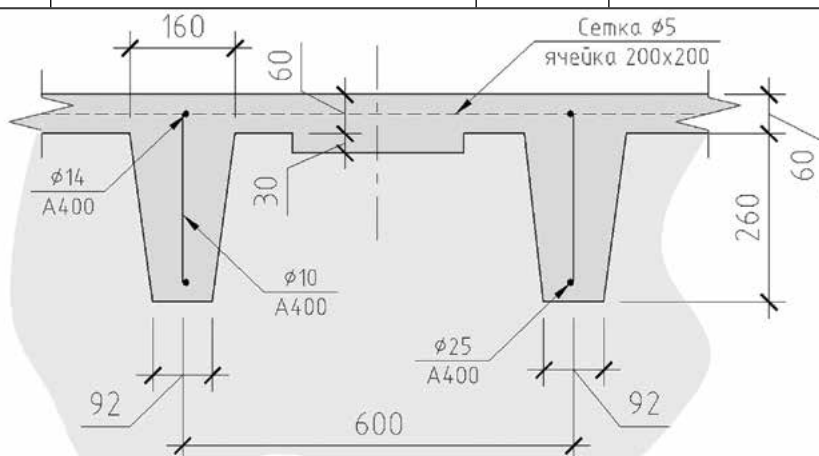
Рис. 1. Монолитное перекрытие
