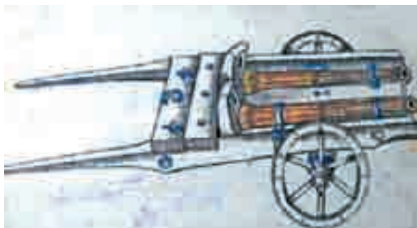
Tunuri-orgă reprezentate în Manuscrisul de la Sibiu
