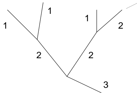
Fig. 2.3.2.1 - Gerarchizzazione secondo Horton Strahler (1957)
