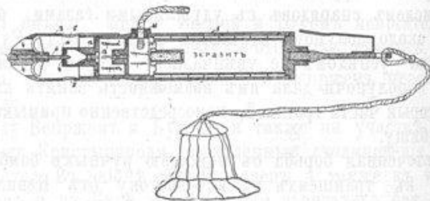
Рис. 4. Ручная бомбочка съ парашютомъ.
