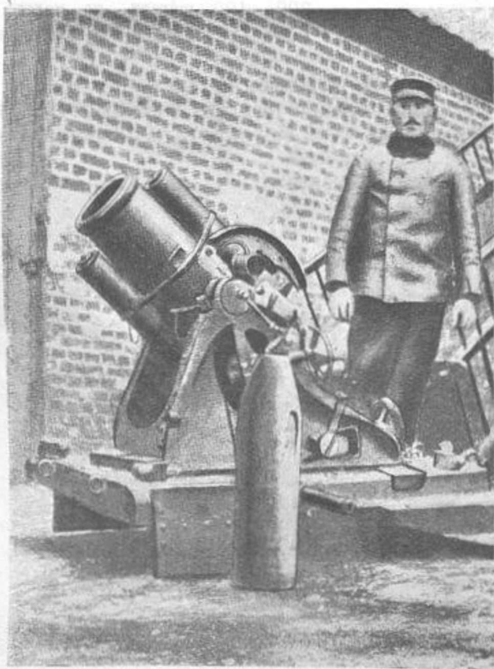
Рис. 14. Тяжелый германскій минометъ.
