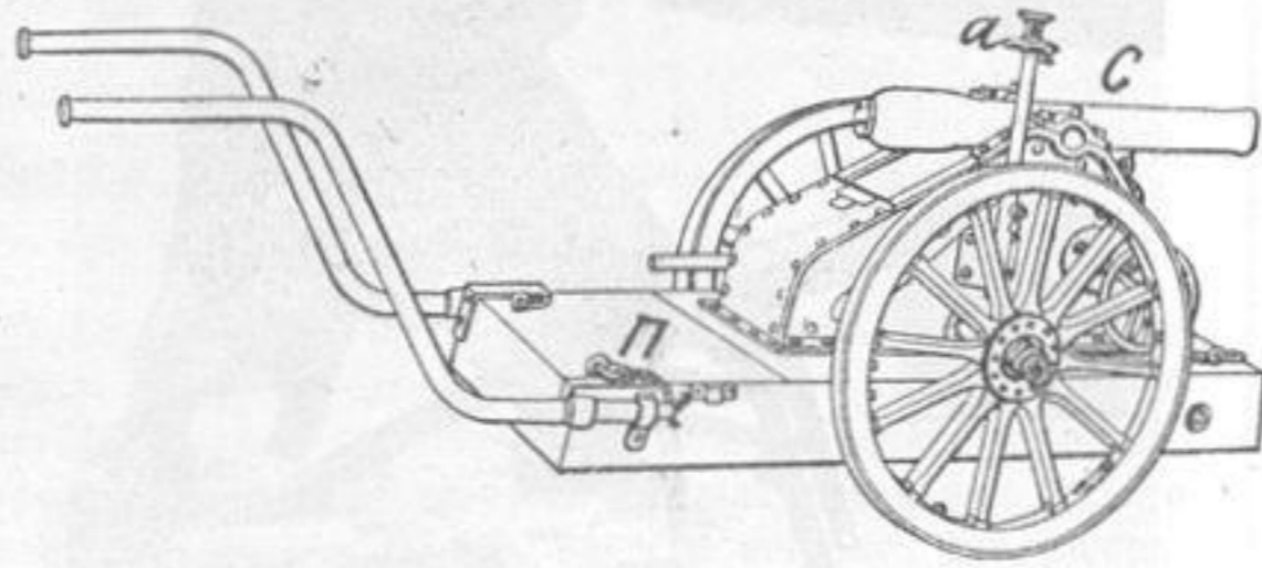
Рис. 12. Бомбометъ Круппа на лафетѣ.
