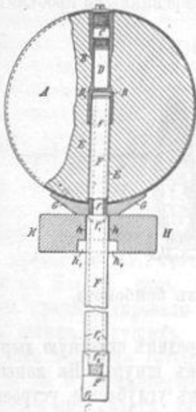
Рис. 13. Бомба къ бомбомету Круппа.
