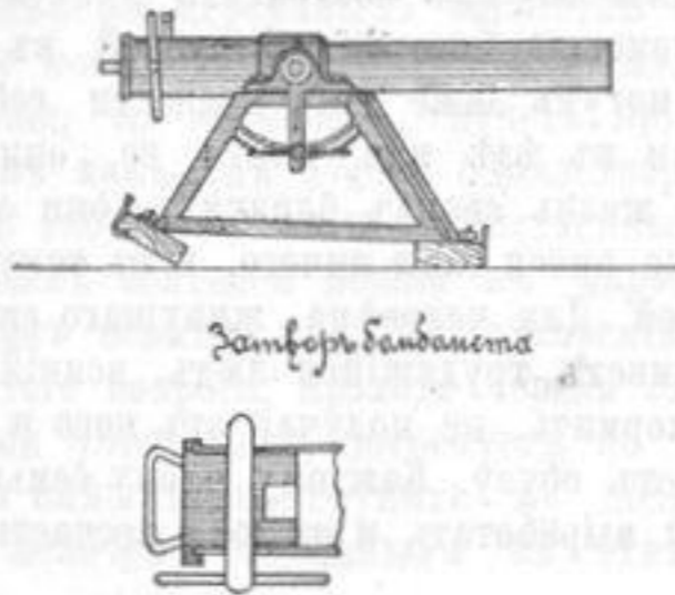
Рис. 7. Пороховой бомбометъ.
