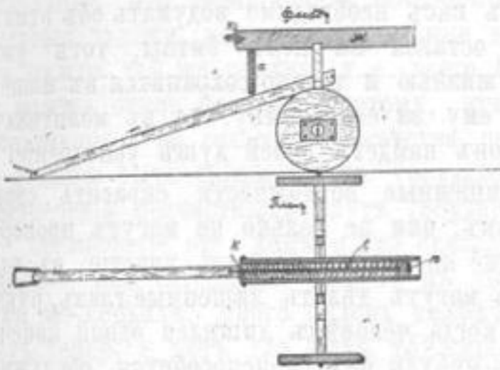
Рис. 6. Пружинный бомбометъ.
