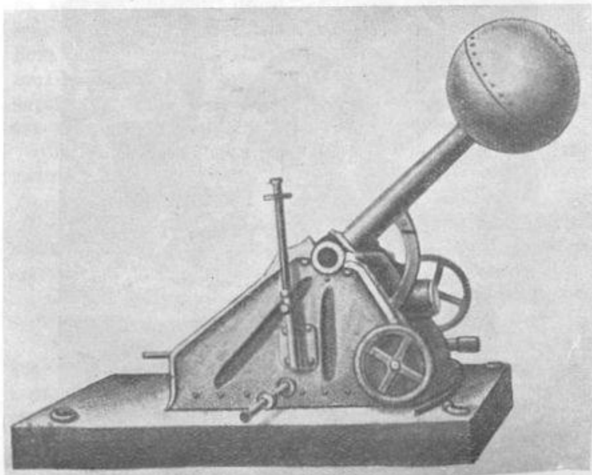
Рис. 11. Бомбометъ завода Круппа.
