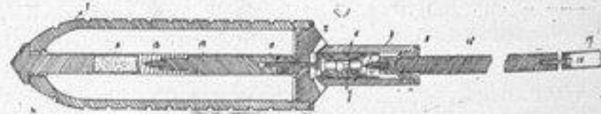
Рис. 5. Австрійская ружейная граната.
