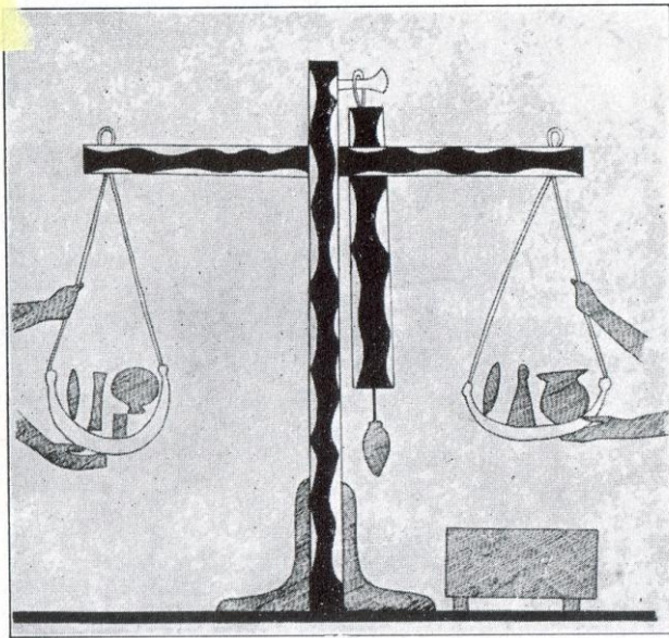
Abb. 49. Anderer Bau einer ägyptischen Waage. Am Wägebalken ein nach unten gerichteter Zeigebalken mit Lot, das gegen eine jedenfalls am Standfuß angebrachte Marke einspielen muß.
