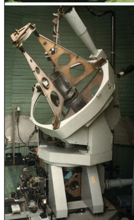
Лазерна станція «Київ» (верхнє фото) і лазерний віддалемір
