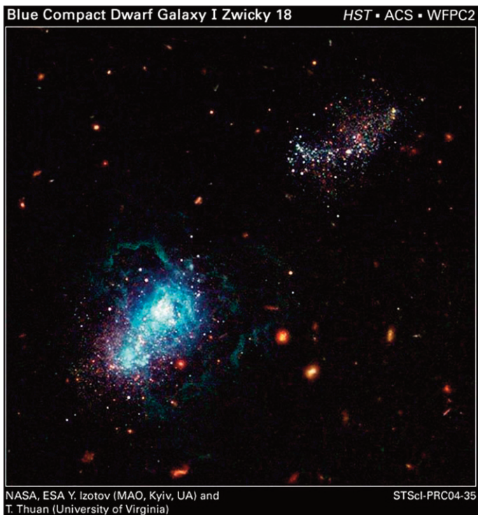
Фото голубої компактно карликової галактики I Zw 18, отримане Ю.І. Ізотовим з допомогою Космічного телескопа імені Габбла
