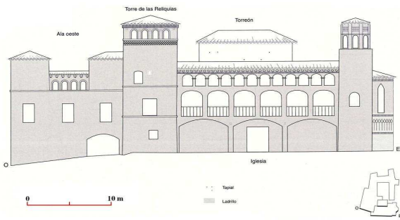
Alzado de la fachada S, hacia 1650 ↑ Planta baja del complejo en 1958 →
